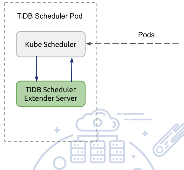
Figure 8: TiDB Scheduler 工作原理
