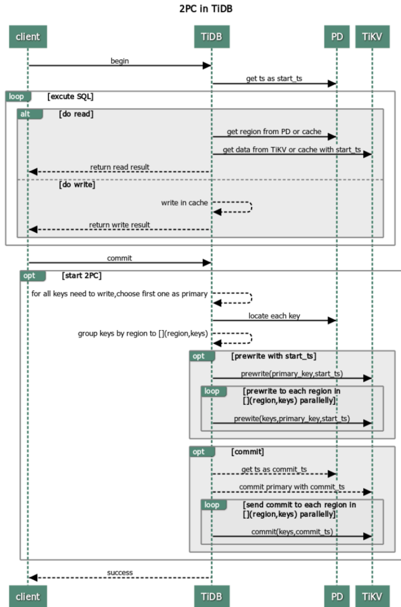
图 219: TiDB 中的两阶段提交
