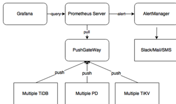
图 18: Prometheus in TiDB
