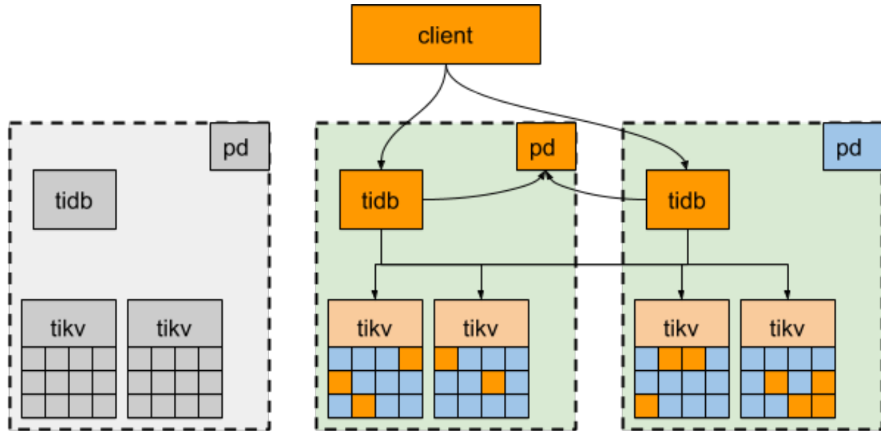
图 13: 三中心部署容灾
