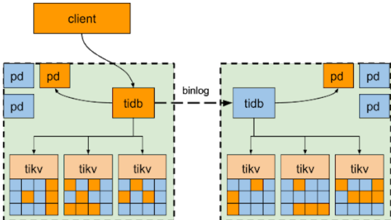
图 16: binlog 同步部署方案
