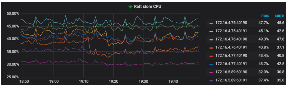
图 265: 图 2 查看 Raftstore CPU
