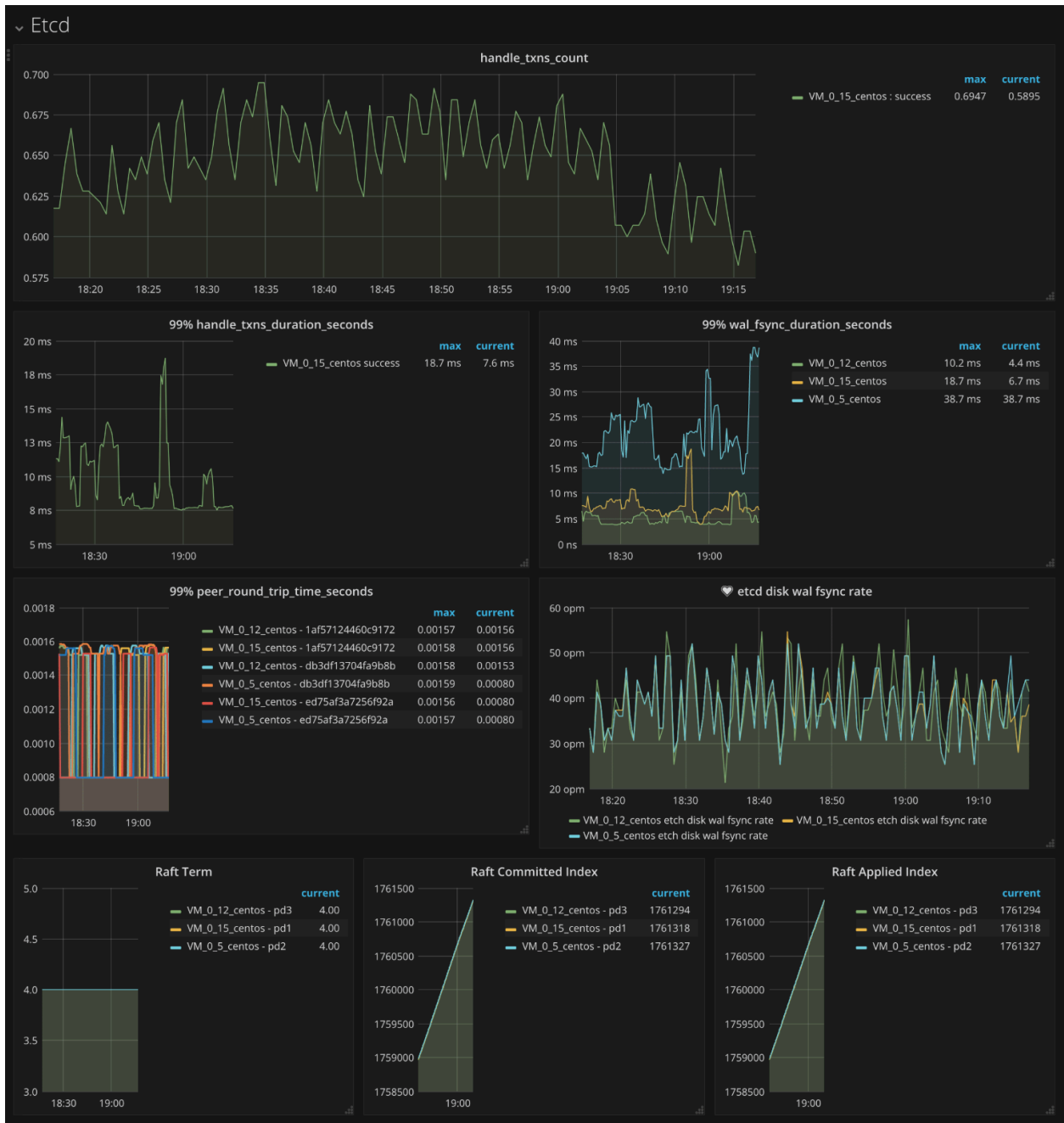
图 228: PD Dashboard - etcd metrics
