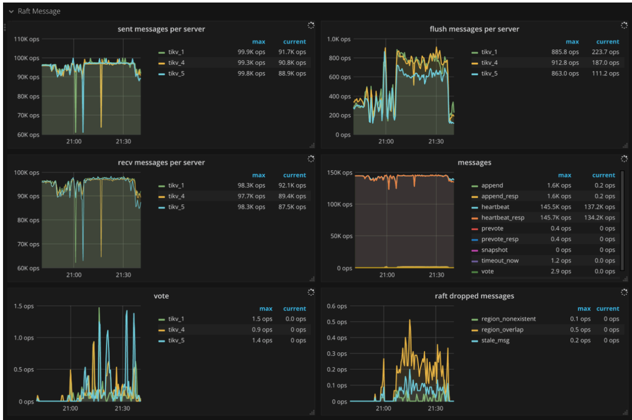
图 236: TiKV Dashboard - Raft message metrics
