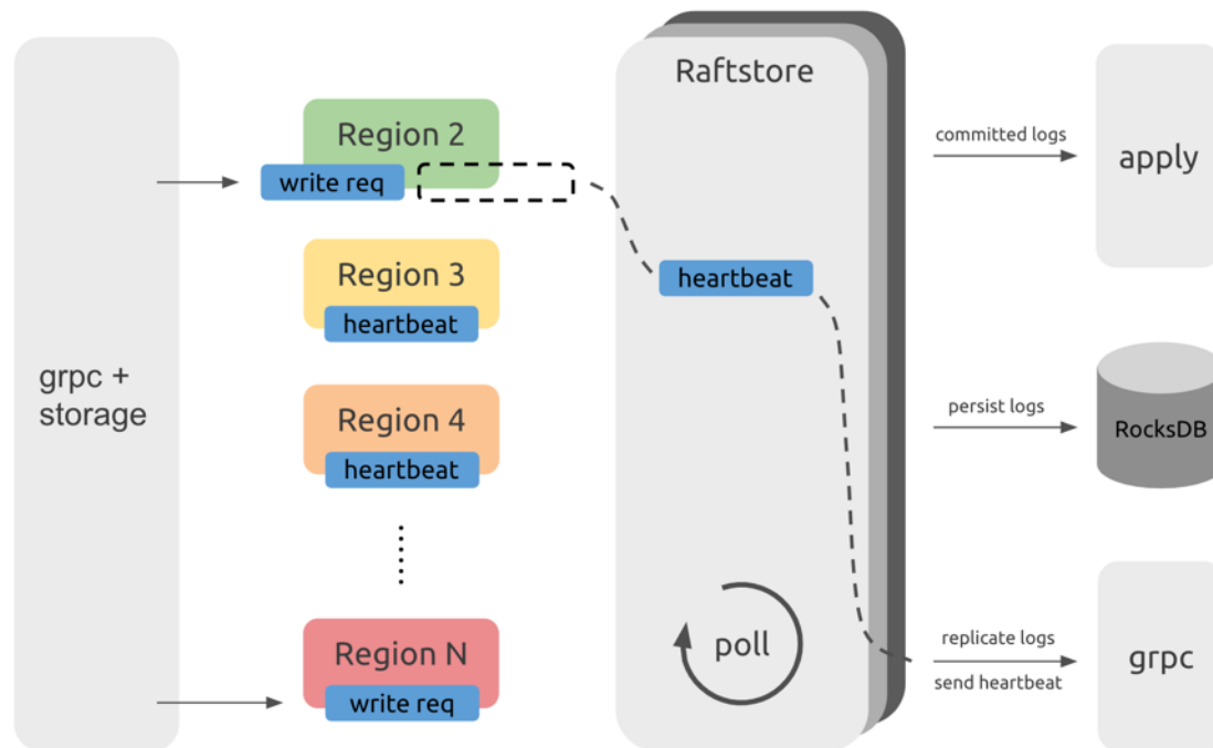
图 264: 图 1 Raftstore 处理流程示意图
