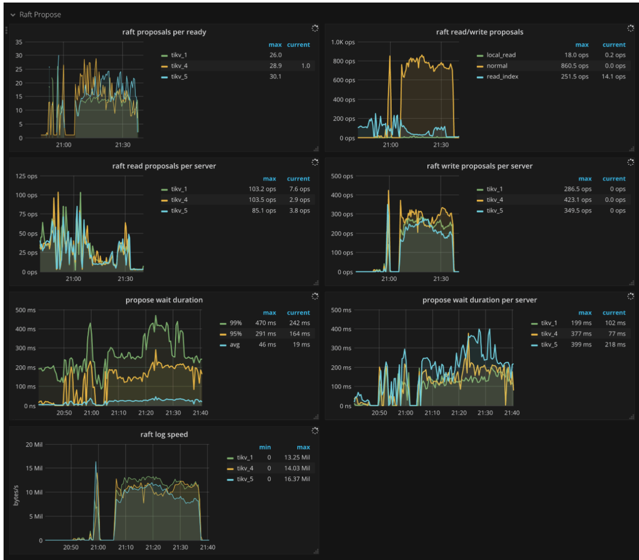
图 237: TiKV Dashboard - Raft propose metrics
