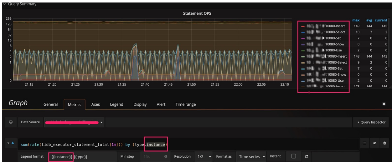
图 252: 给表达式增加一个 instance 维度
