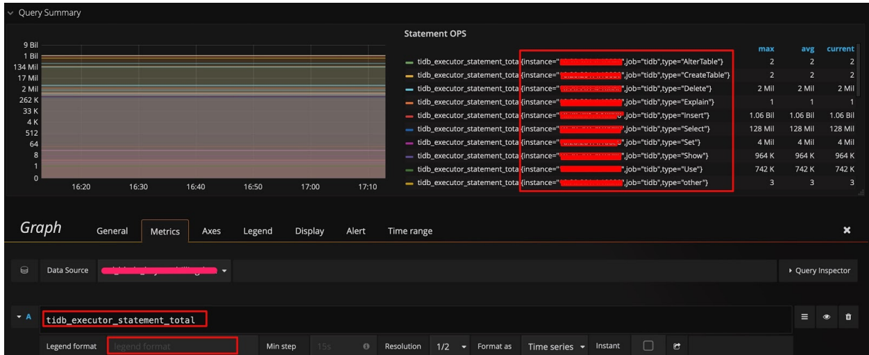
图 251: 编辑表达式并查看所有维度
