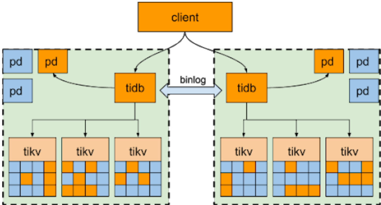
图 17: 两中心 binlog 相互备份方案
