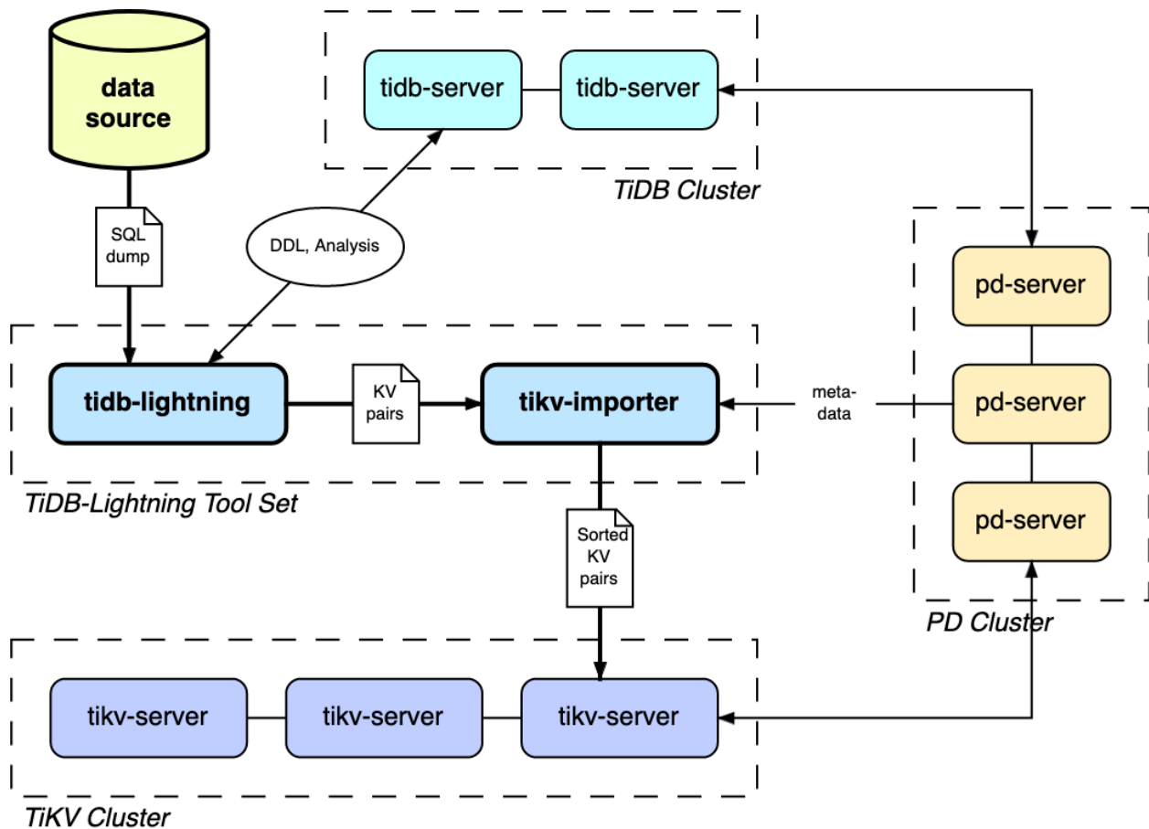
图 26: TiDB Lightning 整体架构
