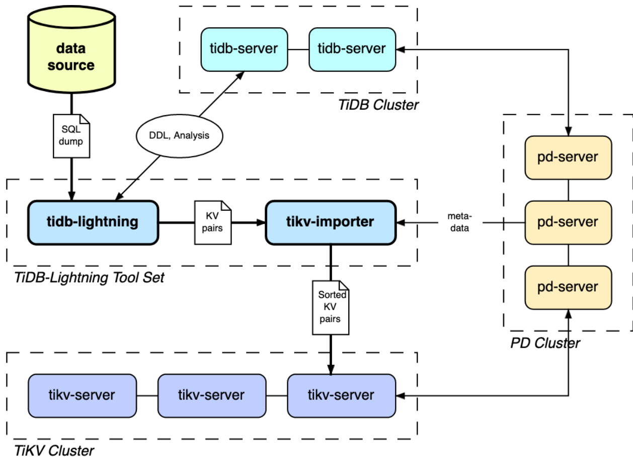
图 336: TiDB Lightning 整体架构
