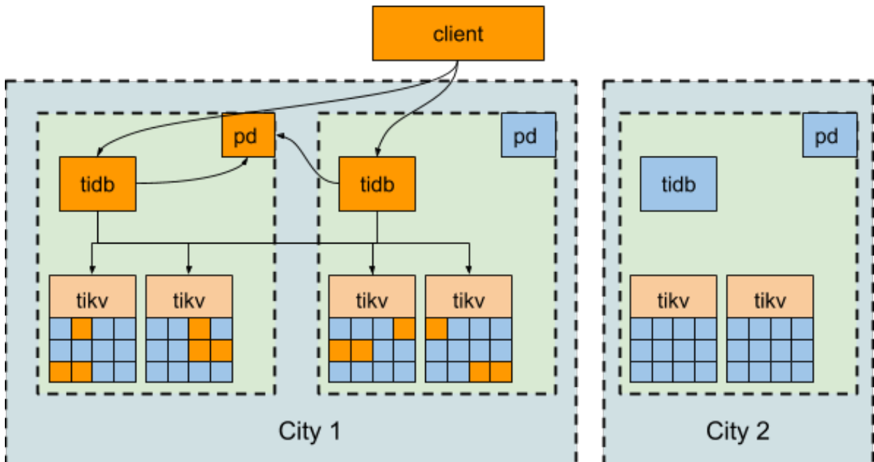
图 30: 两地三中心部署方案
