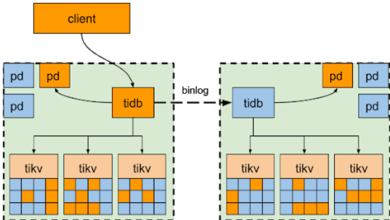
图 31: binlog 同步部署方案
