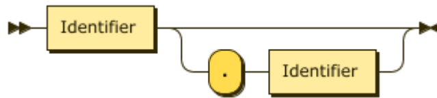
图 55: TableName
