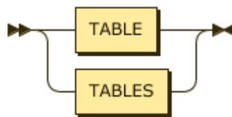
图 112: TableOrTables
