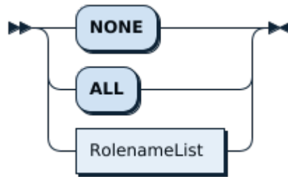
图 205: SetDefaultRoleOpt
