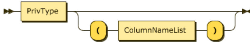
图 176: PrivElem
