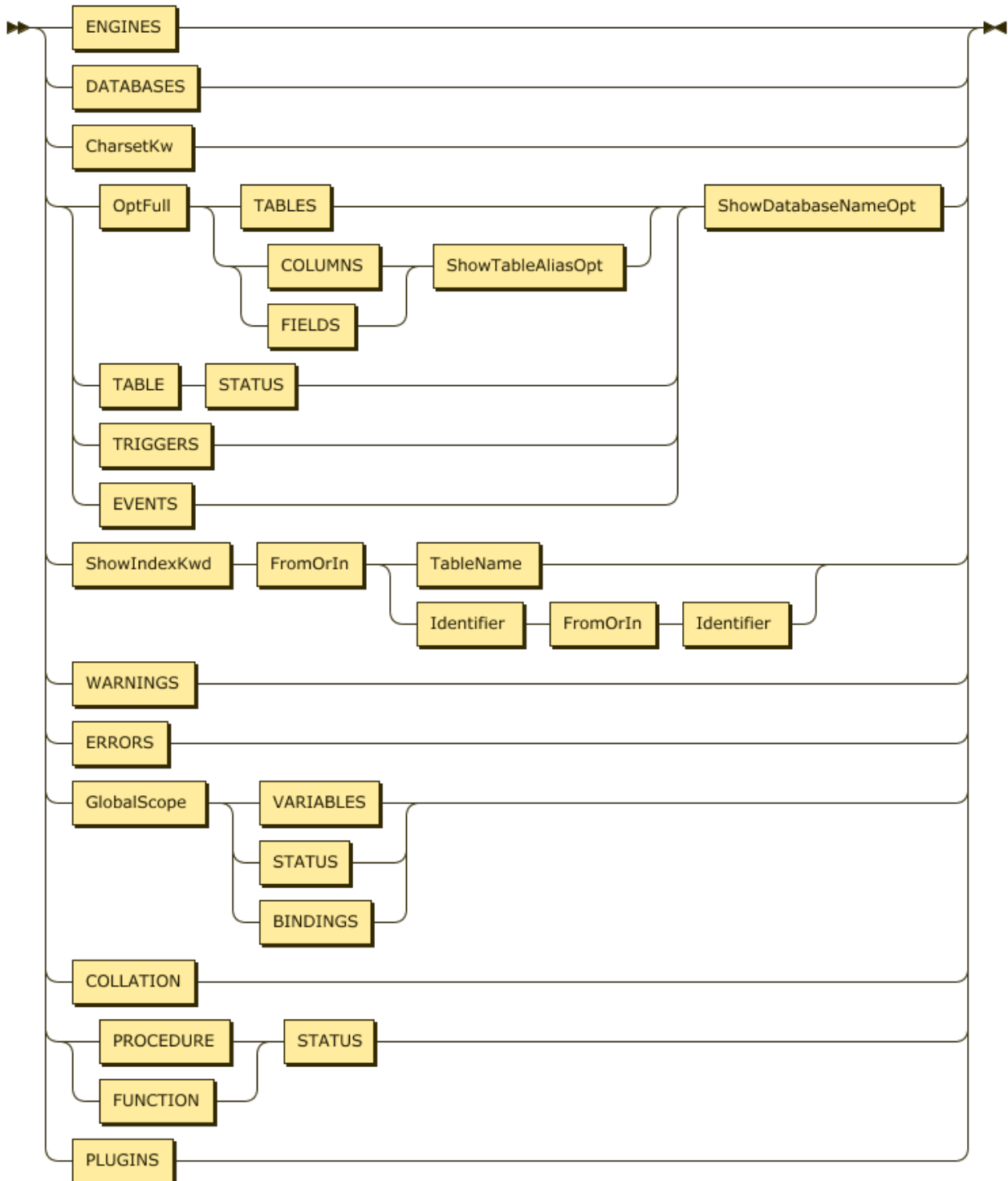
图 242: ShowTargetFilterable
