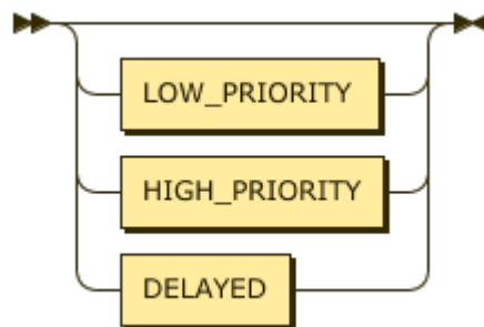
图 151: PriorityOpt
