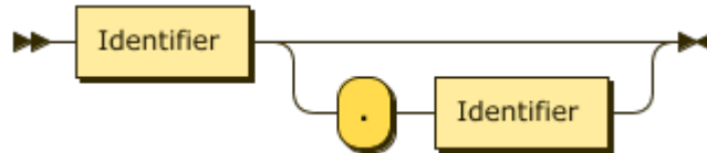
图 259: TableName
