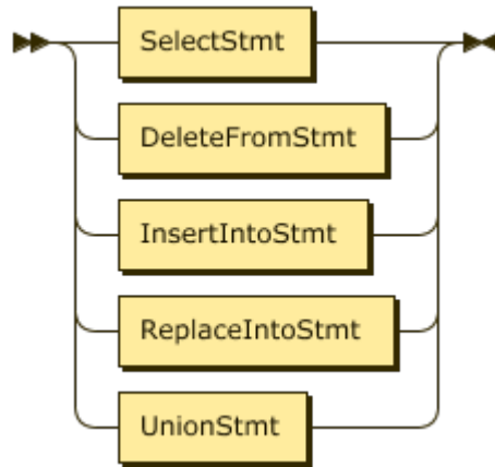
图 123: ExplainableStmt
