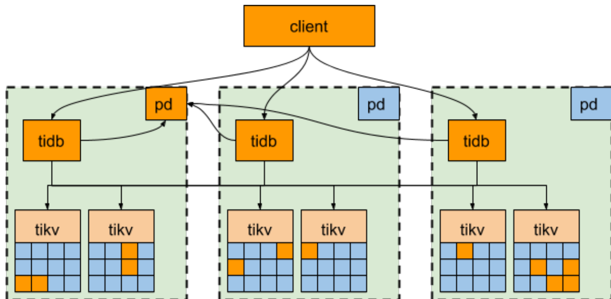
图 27: 三中心部署
