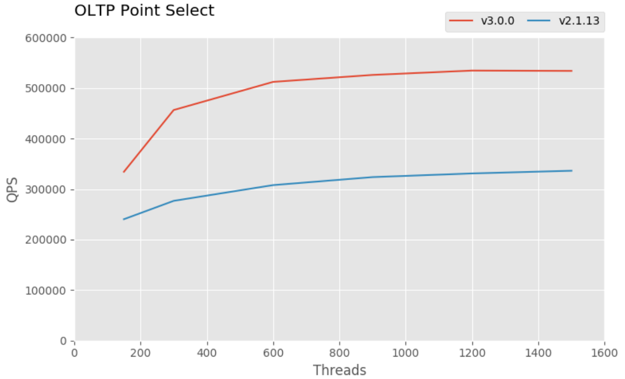
图 4: point select
