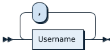
图 183: UsernameList
