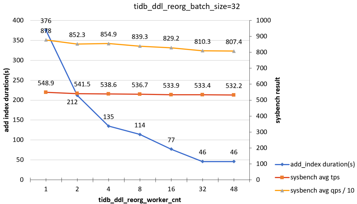
图 17: add-index-load-2-b32
