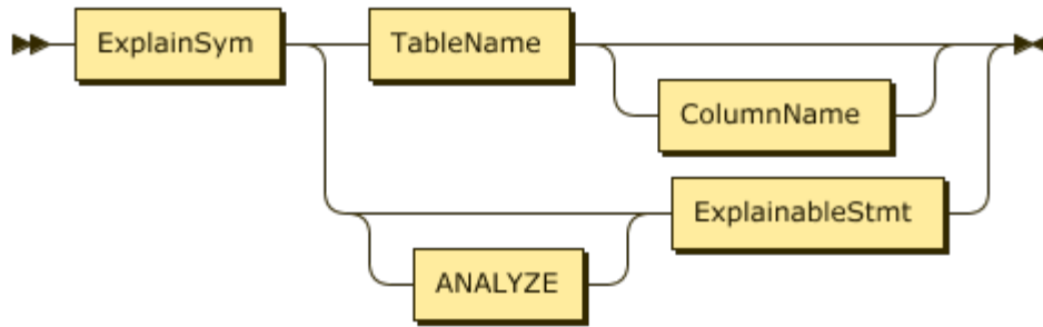
图 125: ExplainStmt
