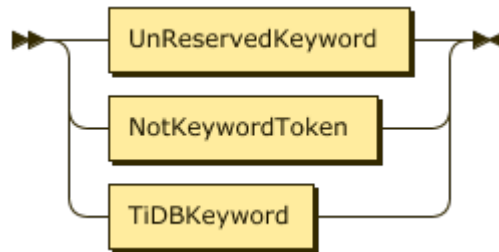
图 108: Identifier
