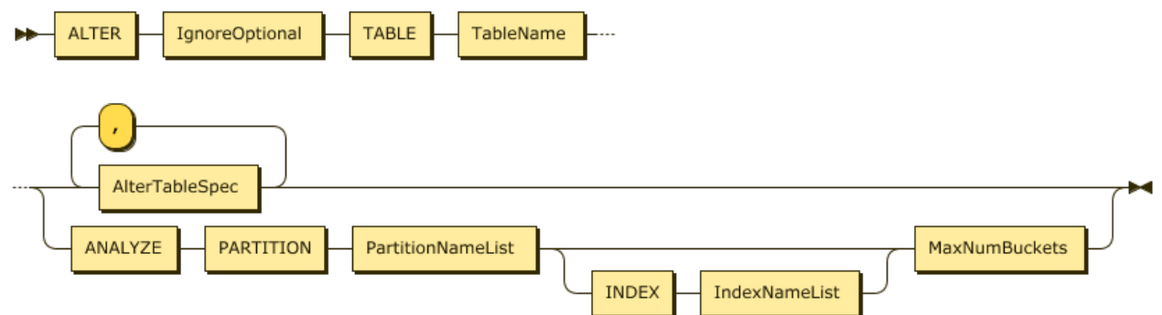
图 97: AlterTableStmt
