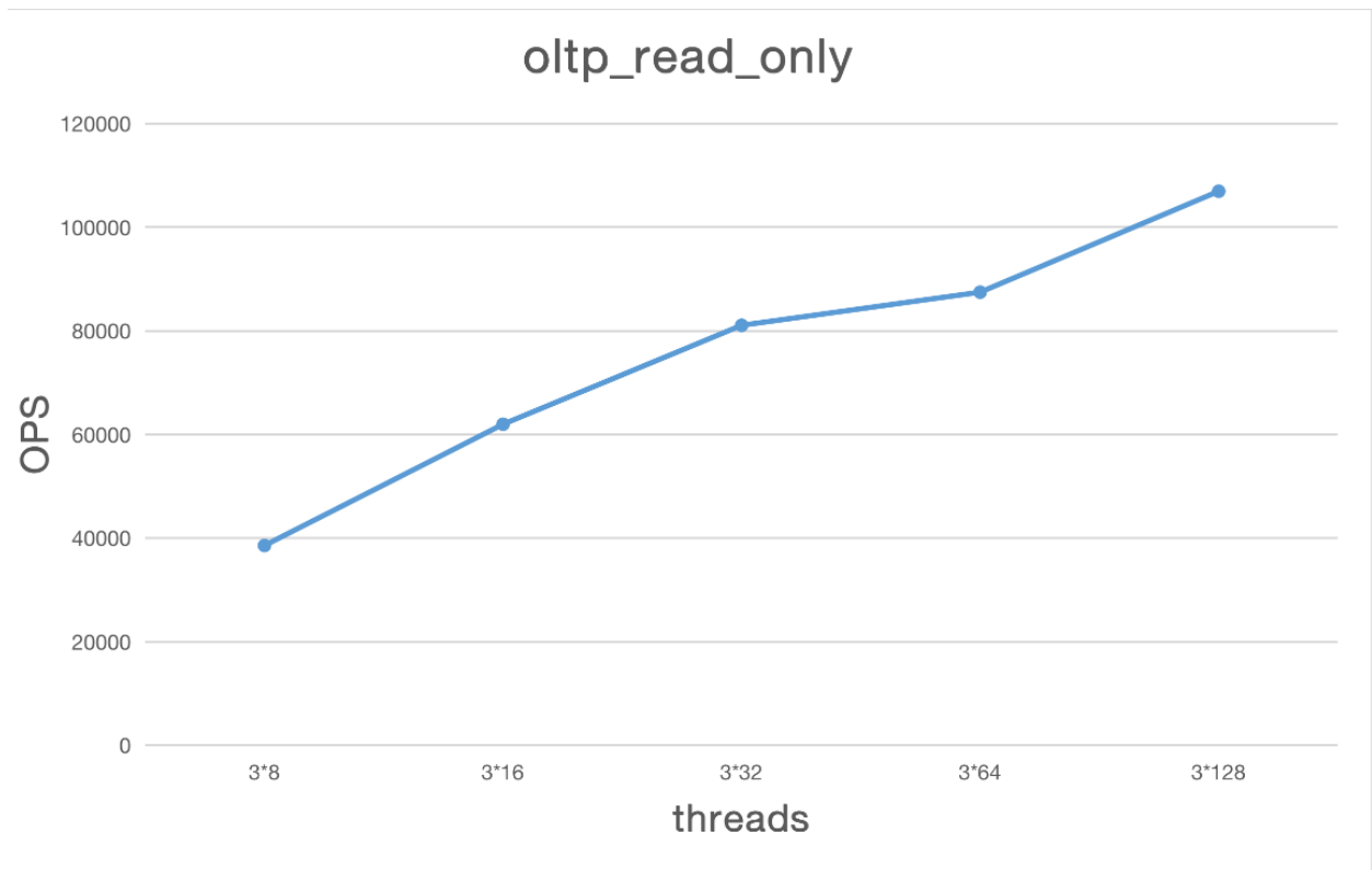
图 3: oltp_read_only
