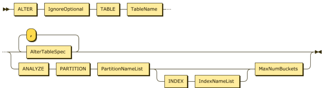
图 159: AlterTableStmt
