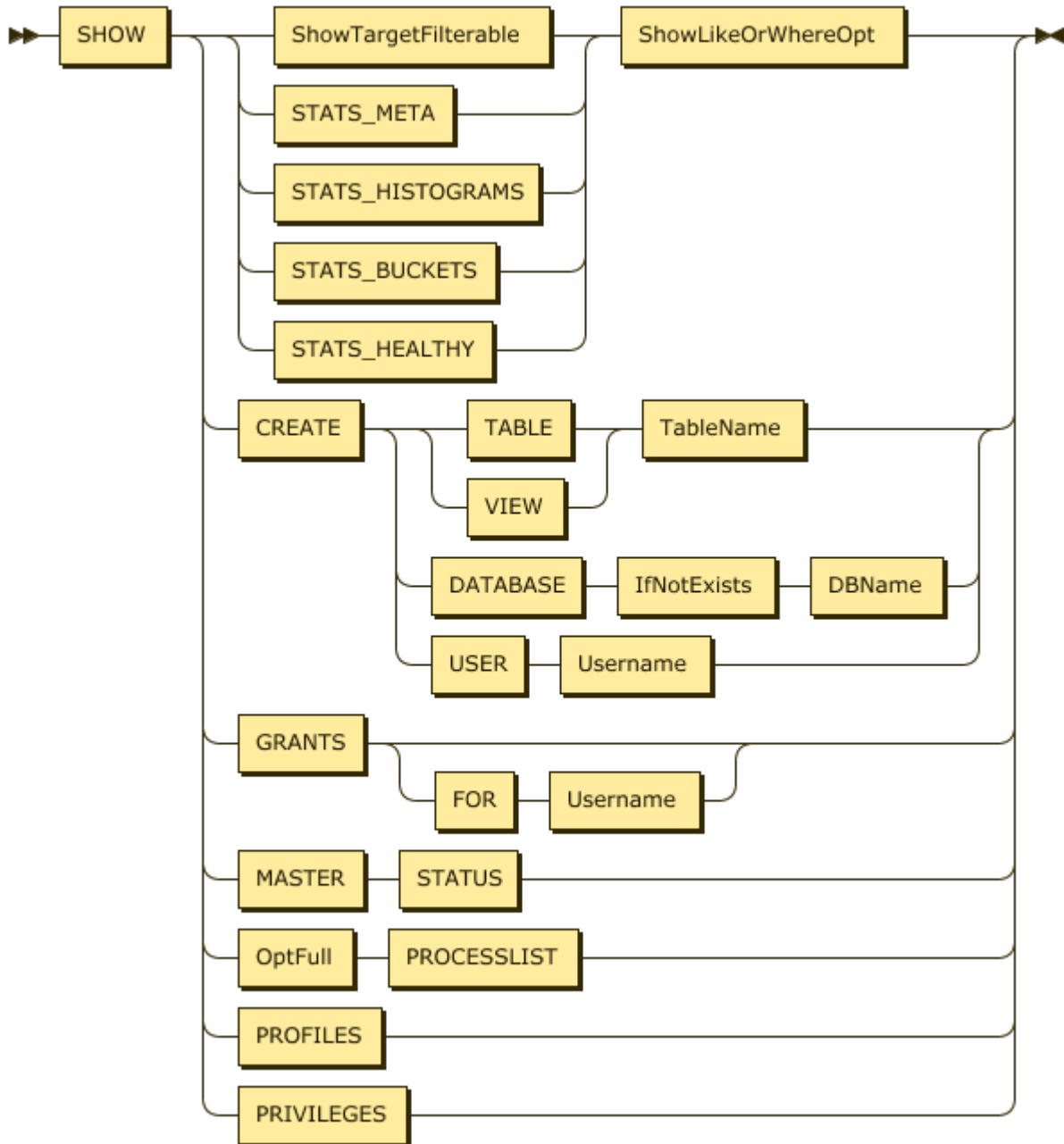
图 241: ShowStmt
