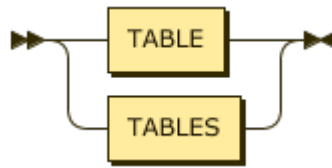
图 137: TableOrTables
