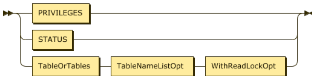
图 133: FlushOption
