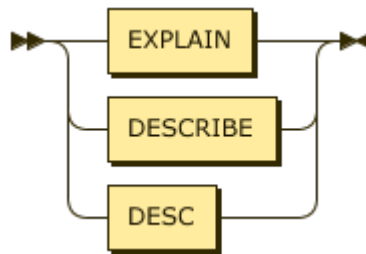
图 121: ExplainSym
