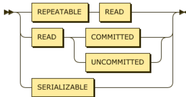
图 208: IsolationLevel
