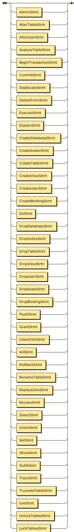
图 184: Statement 369
