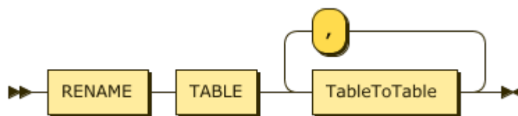
图 167: RenameTableStmt
