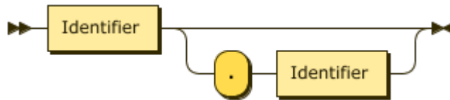
图 154: TableName
