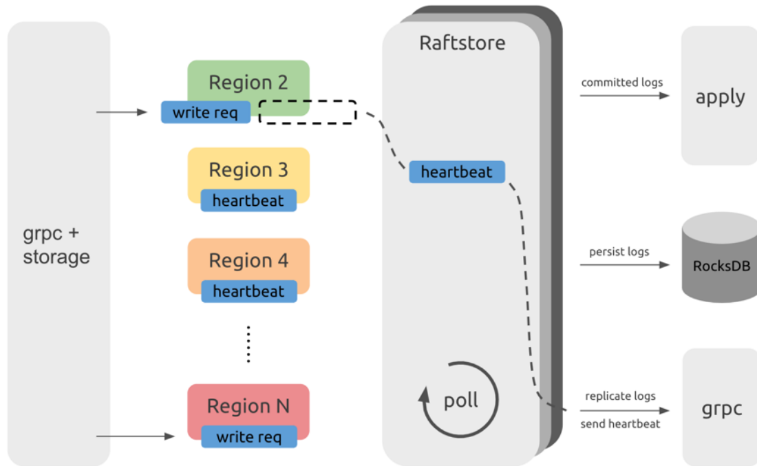
图 324: 图 1 Raftstore 处理流程示意图
