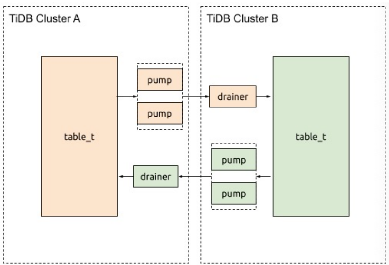
图 331: 使用场景示例图
