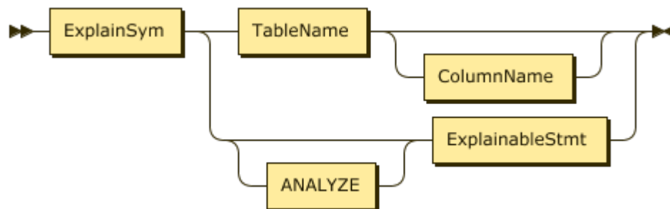
图 122: ExplainStmt
