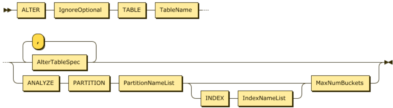
图 165: AlterTableStmt
