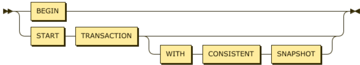
图 252: BeginTransactionStmt
