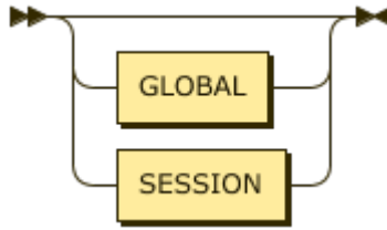
图 240: GlobalScope
