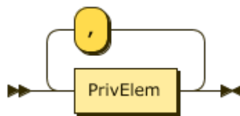
图 141: PrivElemList
