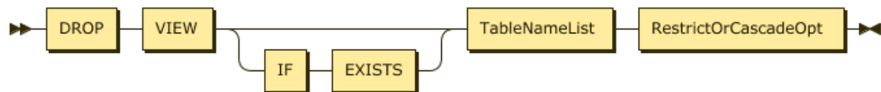
图 116: DropViewStmt
