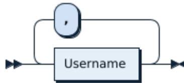
图 200: UsernameList
