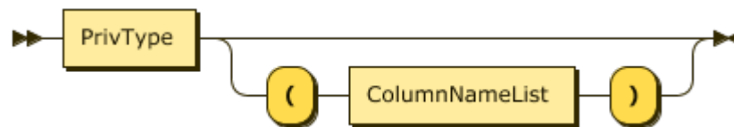
图 142: PrivElem
