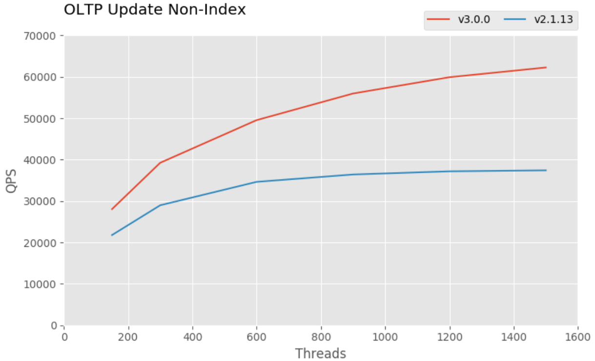
图 5: update non-index
