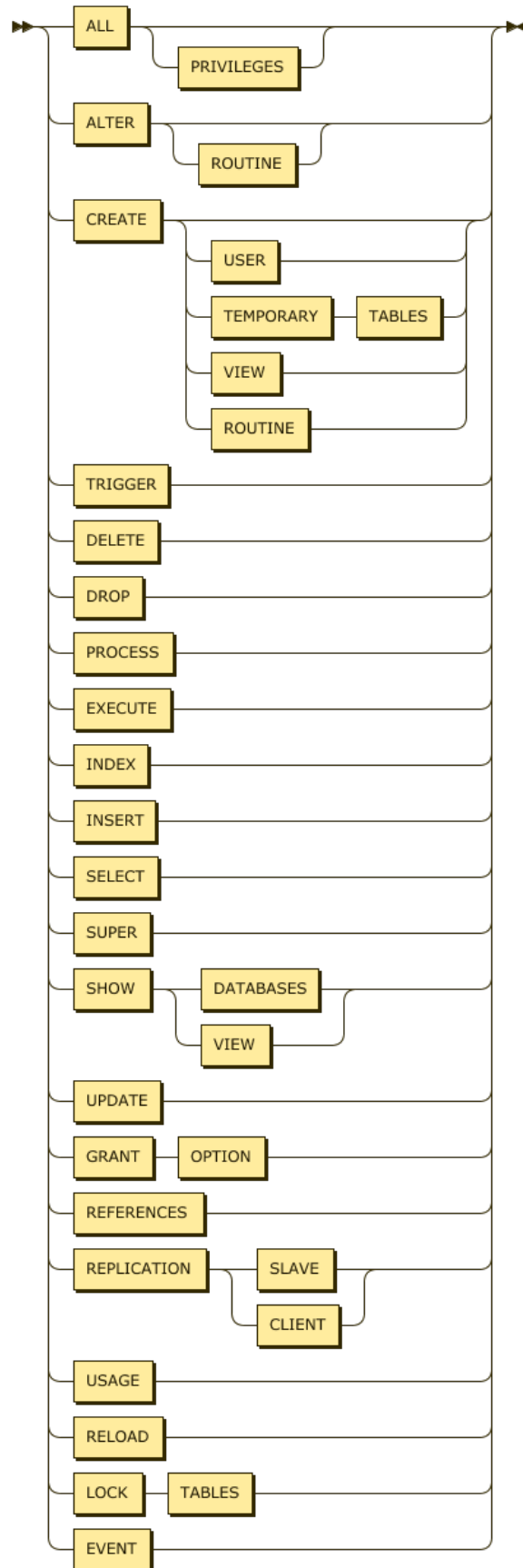
图 177: PrivType 362
