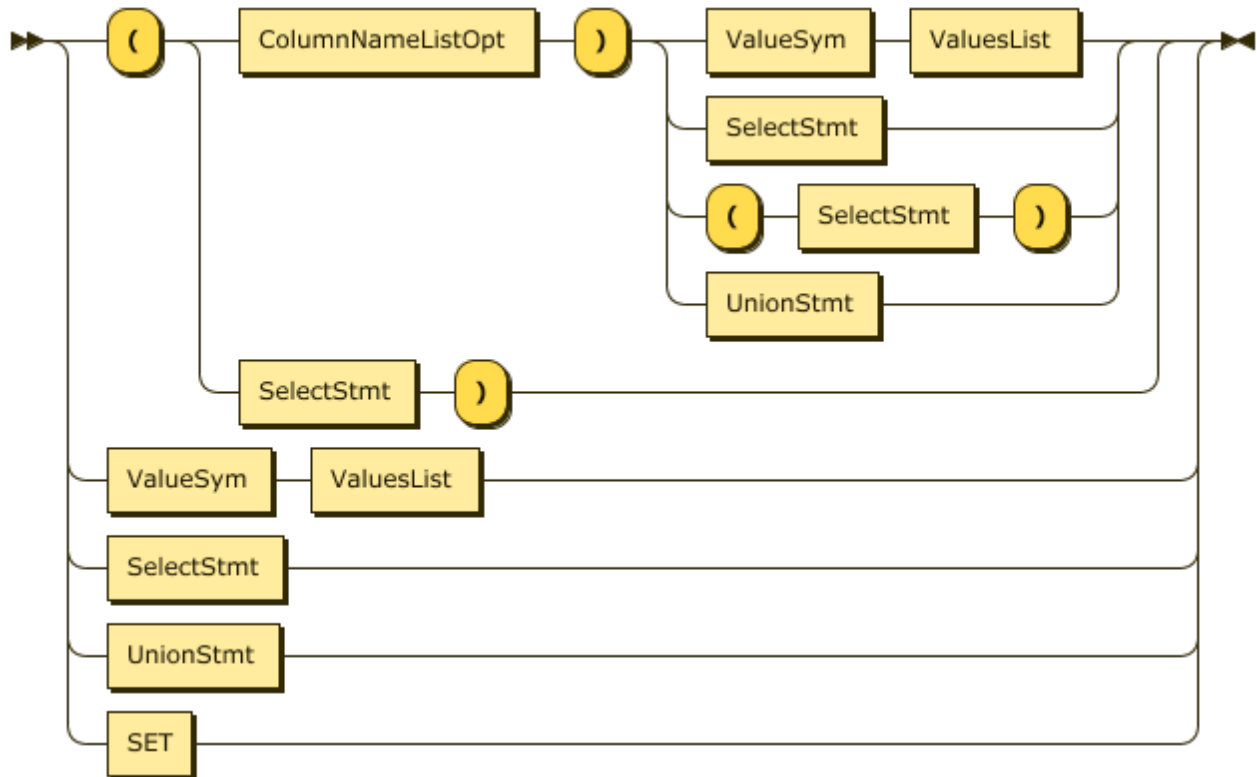
图 155: InsertValues
