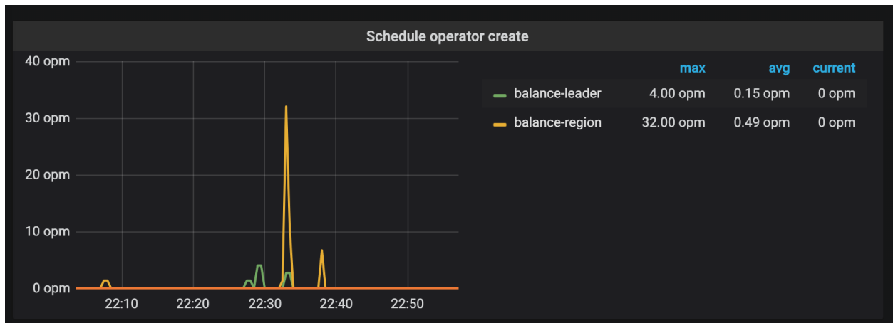
图 303: QPS5
