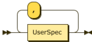
图 78: UserSpecList
