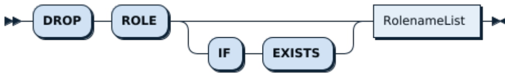
图 109: DropRoleStmt
