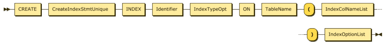
图 51: CreateIndexStmt
