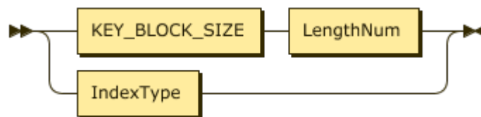
图 58: IndexOption
