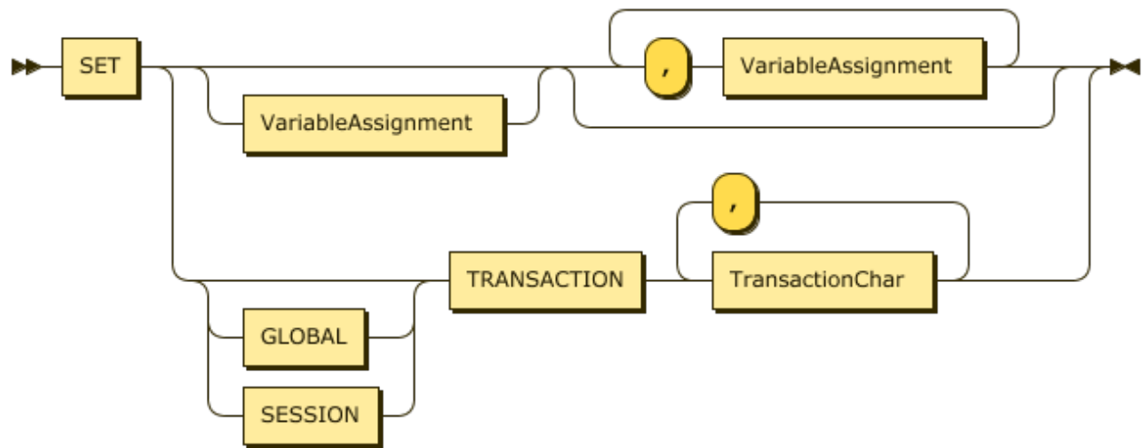
图 209: SetStmt
