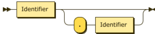
图 67: TableName
