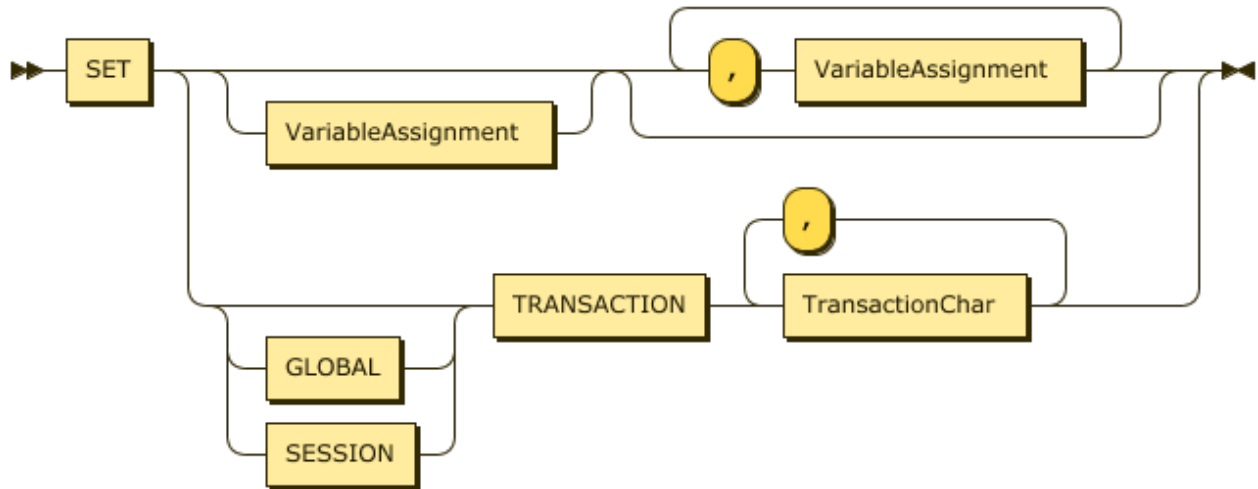
图 206: SetStmt
