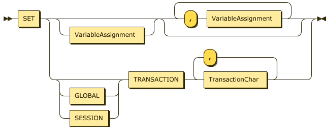
图 202: SetStmt
