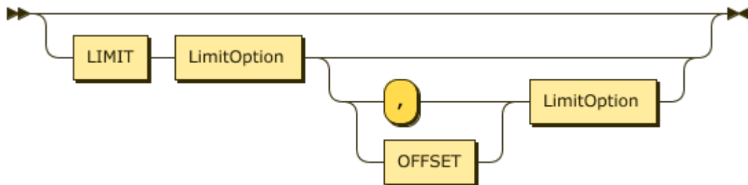
图 195: SelectStmtLimit
