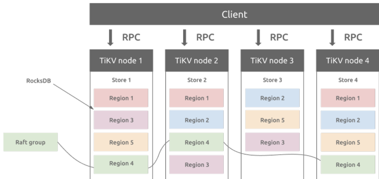
图 329: TiKV 架构
