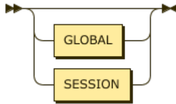
图 249: GlobalScope
