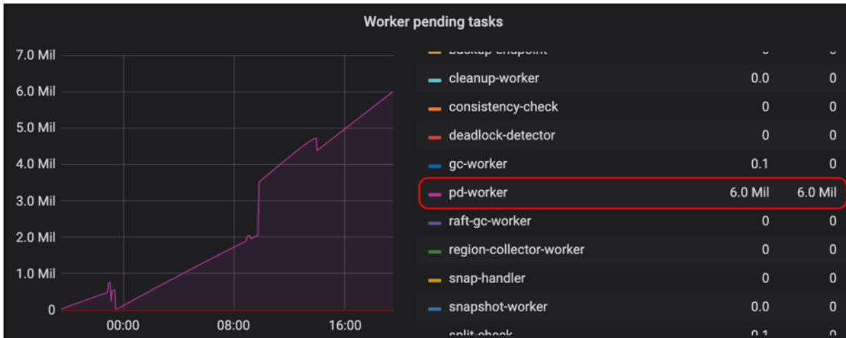
图 327: 图 4 查看 pd-worker
