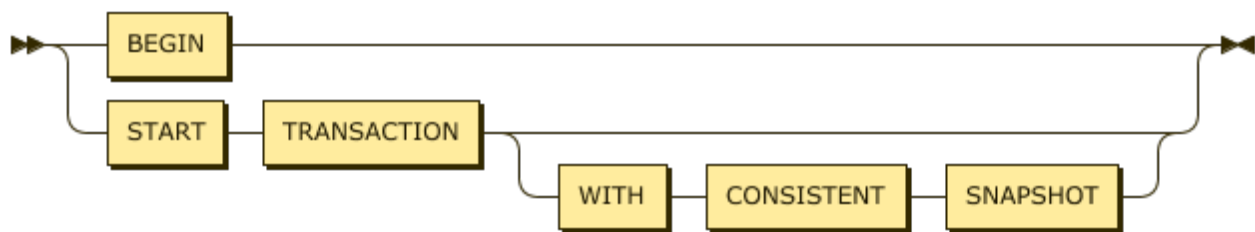
图 38: BeginTransactionStmt
