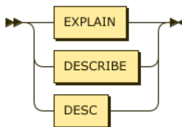
图 124: ExplainSym
