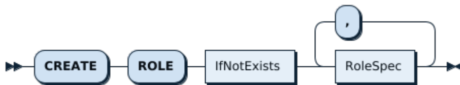
图 59: CreateRoleStmt
