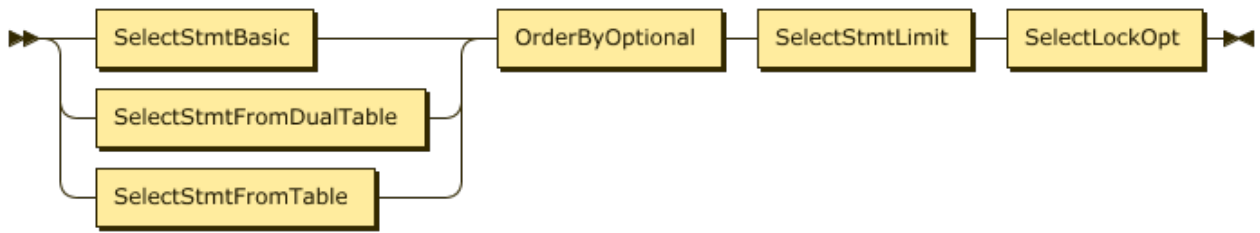
图 185: SelectStmt
