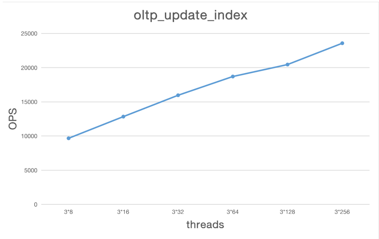
图 2: oltp_update_index
