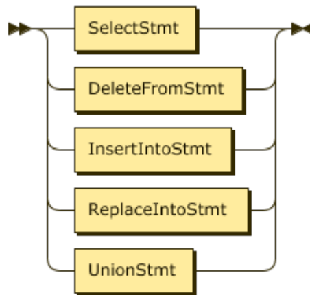
图 126: ExplainableStmt
