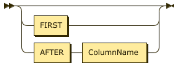
图 163: ColumnPosition
