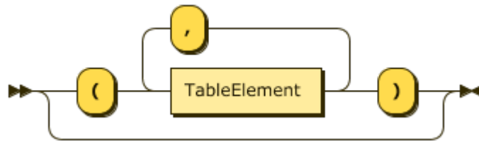
图 68: TableElementListOpt
