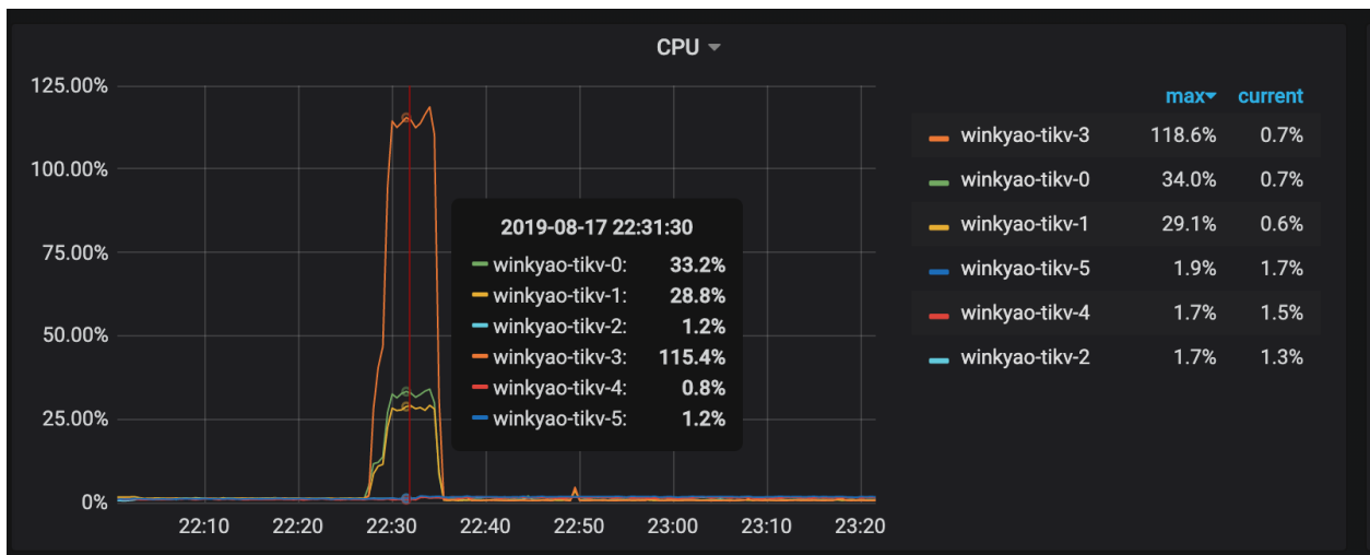
图 299: QPS2
