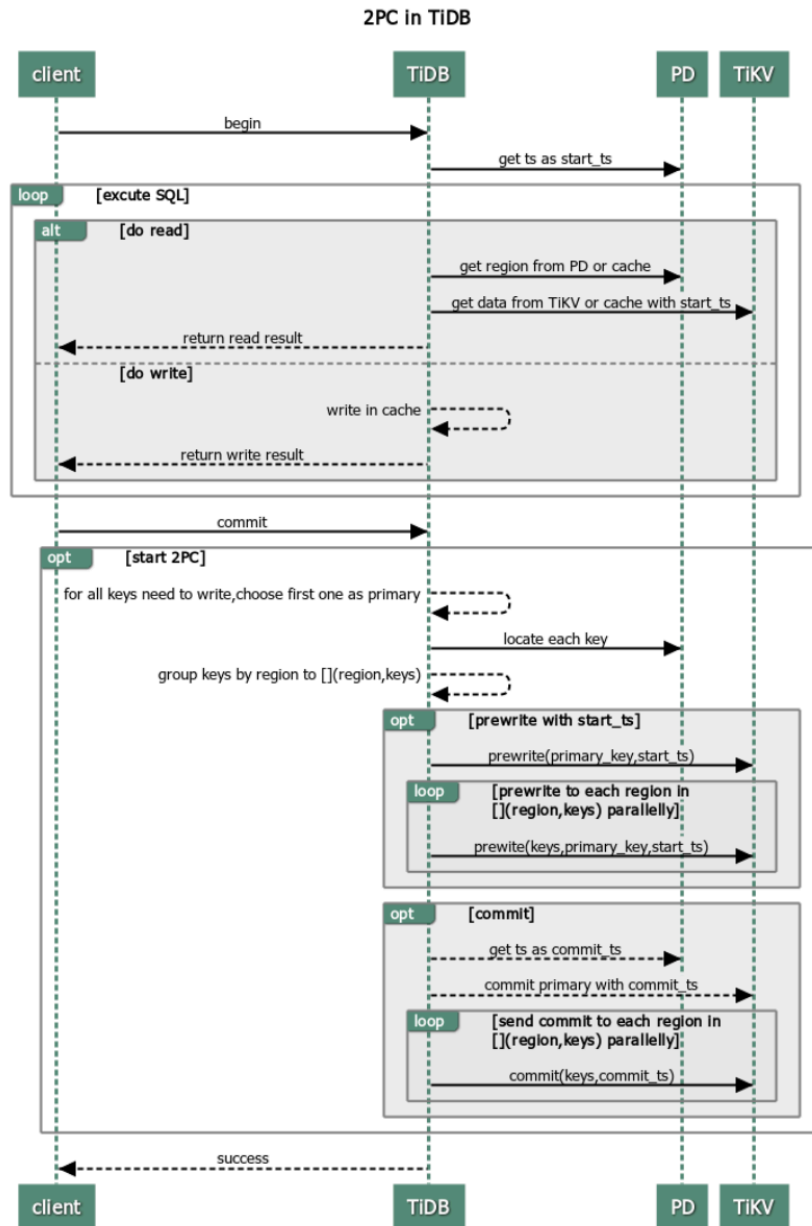
图 267: TiDB 中的两阶段提交
