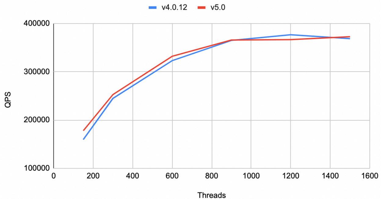
图 1: Point Select
