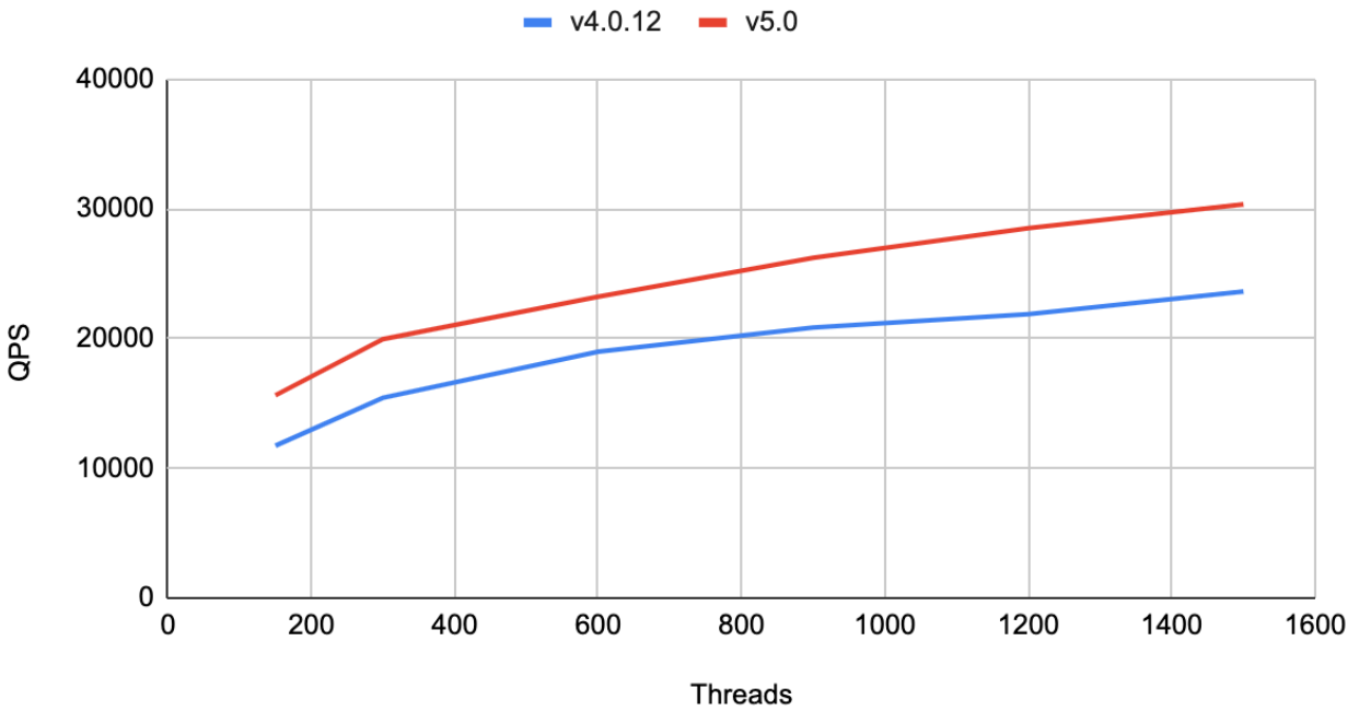
图 3: Update Index
