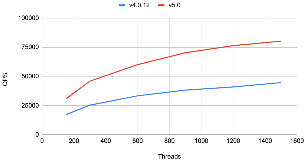
图 2: Update Non-index
