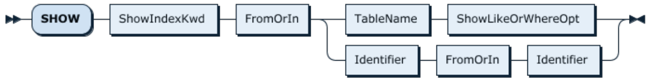
图 281: ShowIndexStmt
