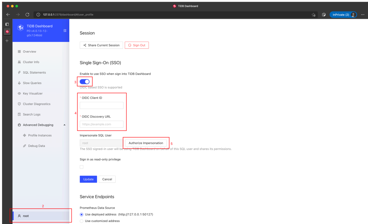
图 449: 操作示例
