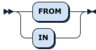
图 312: FromOrIn
