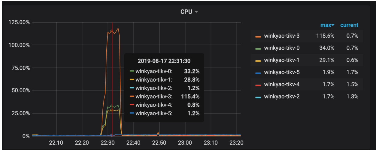
图 84: QPS2
