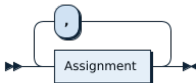
图 341: AssignmentList
