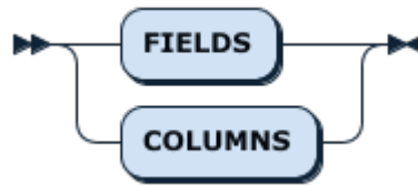
图 257: FieldsOrColumns
