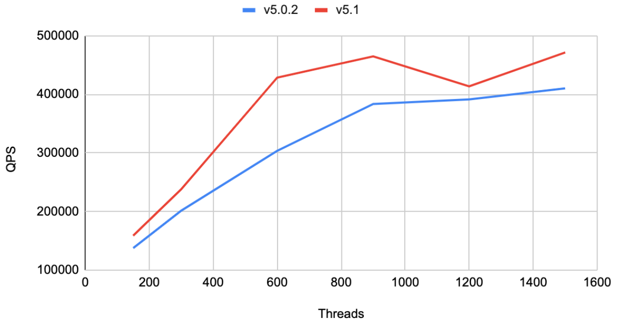
图 1: Point Select
