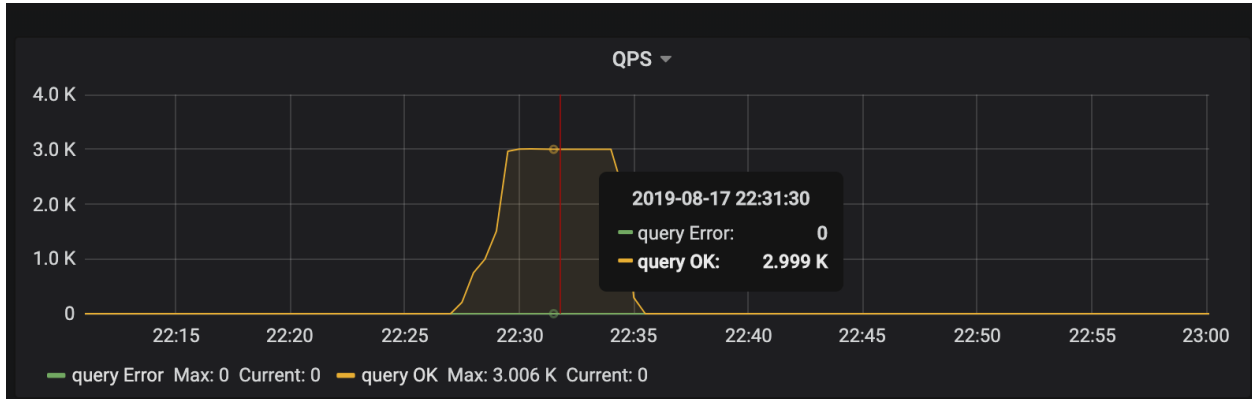
图 83: QPS1
