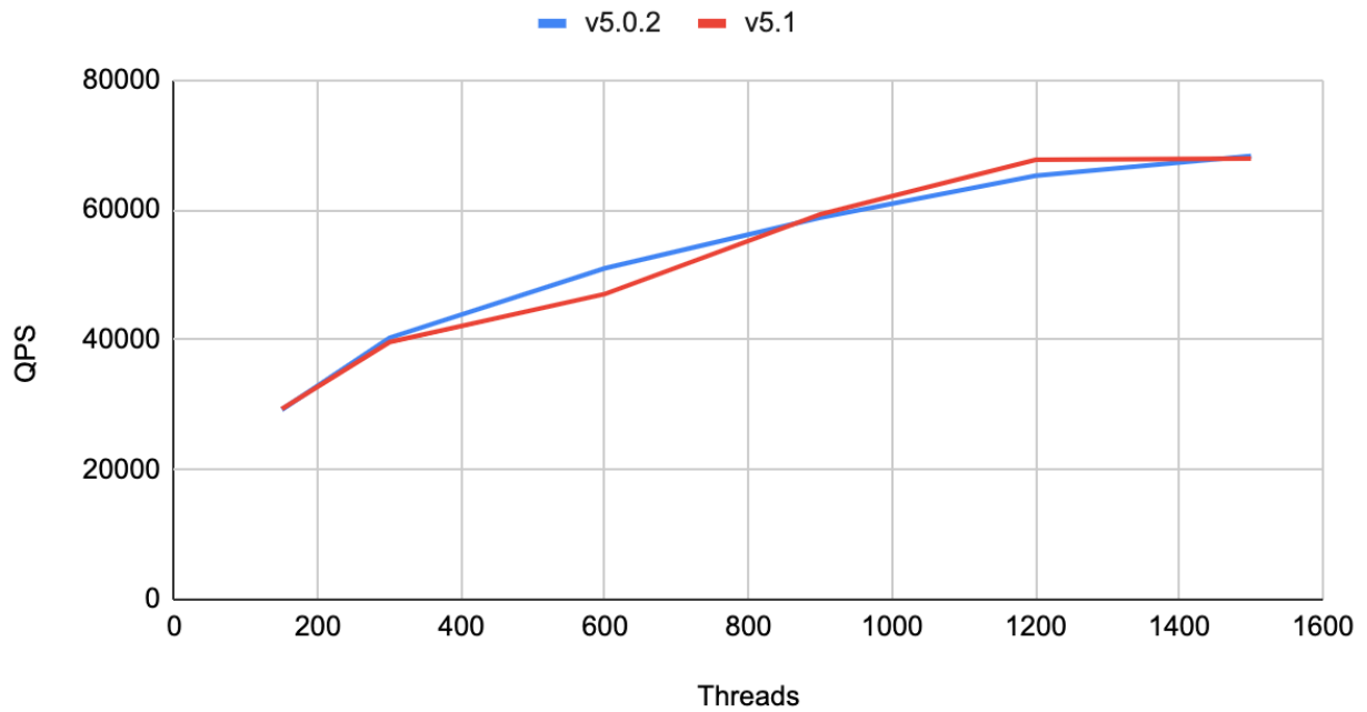
图 2: Update Non-index
