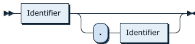
图 325: TableName
