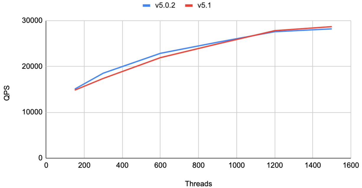
图 3: Update Index
