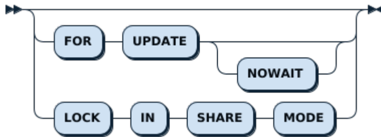
图 225: SelectLockOpt
