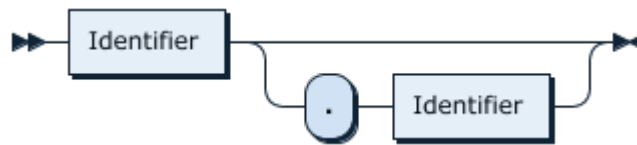
图 267: TableName
