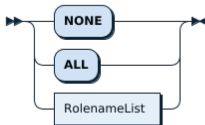
图 228: SetDefaultRoleOpt
