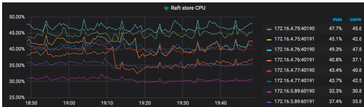
图 113: 图 2 查看 Raftstore CPU
