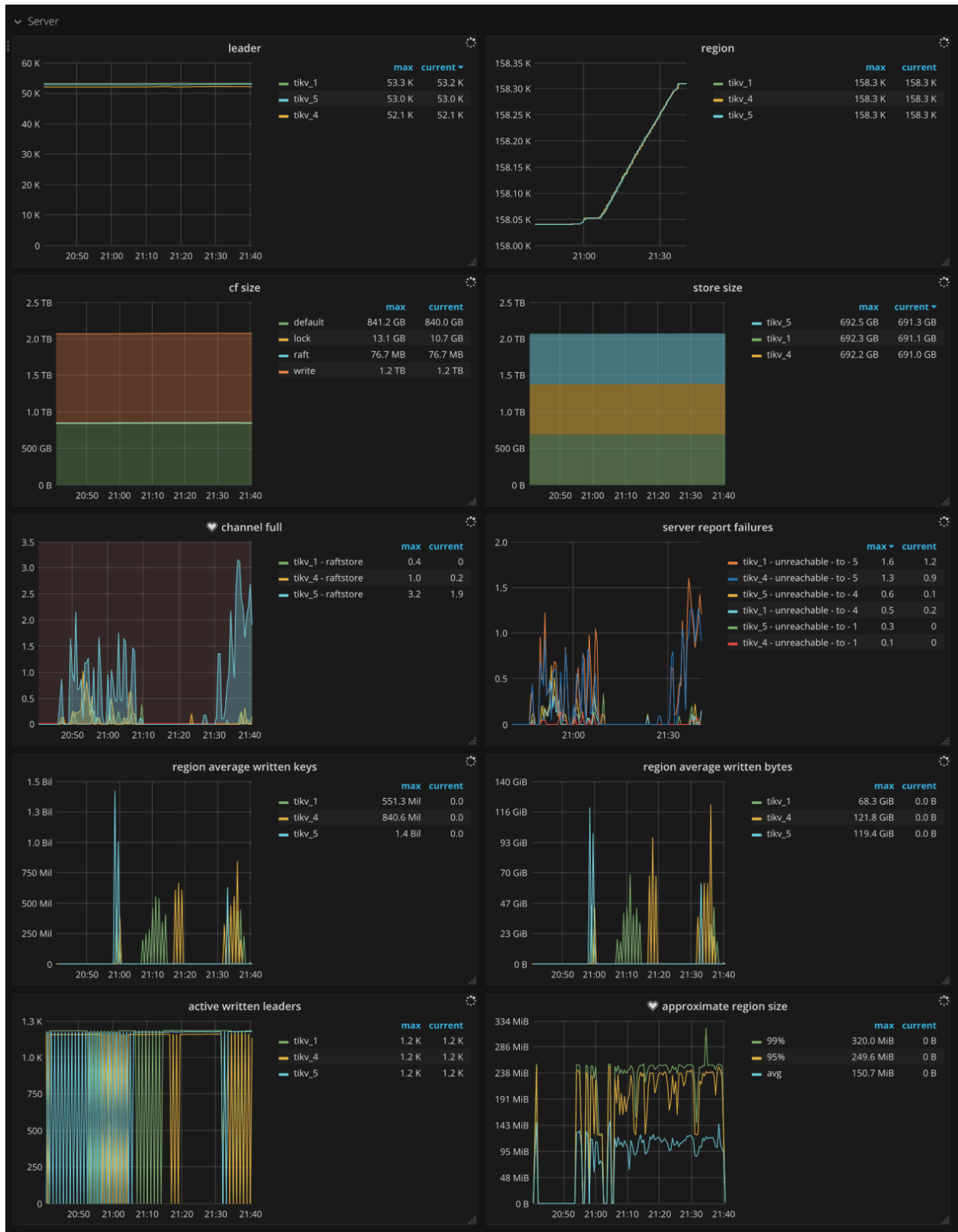
图 203: TiKV Dashboard - Server metrics
