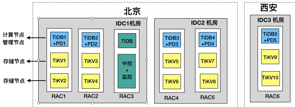
图 79: 两地三中心配置详图
