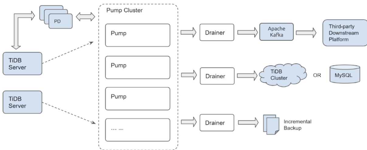
图 160: TiDB Binlog 架构
