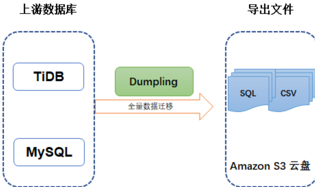
图 122: Dumpling 导出数据
