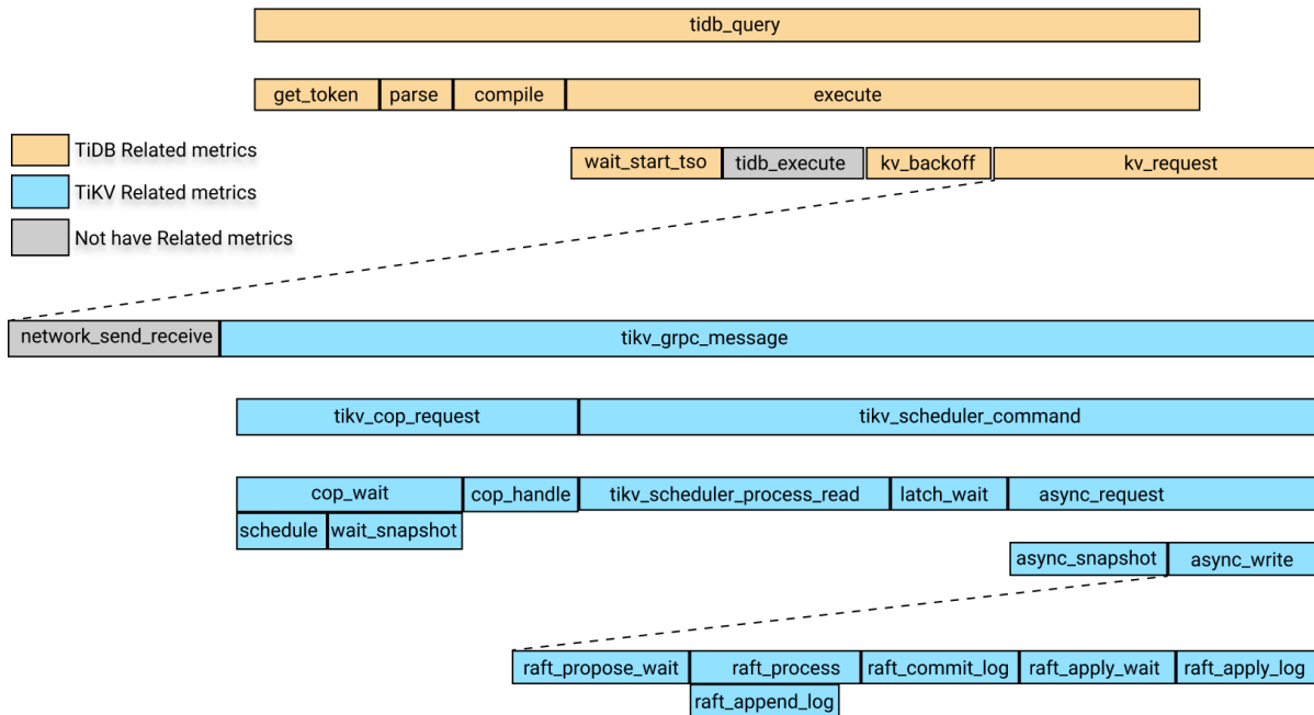
图 420: 各个模块耗时关系图
