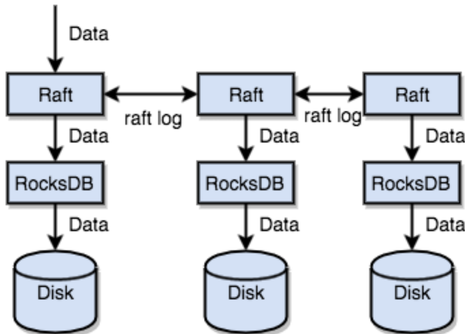
图 173: Raft in TiDB
