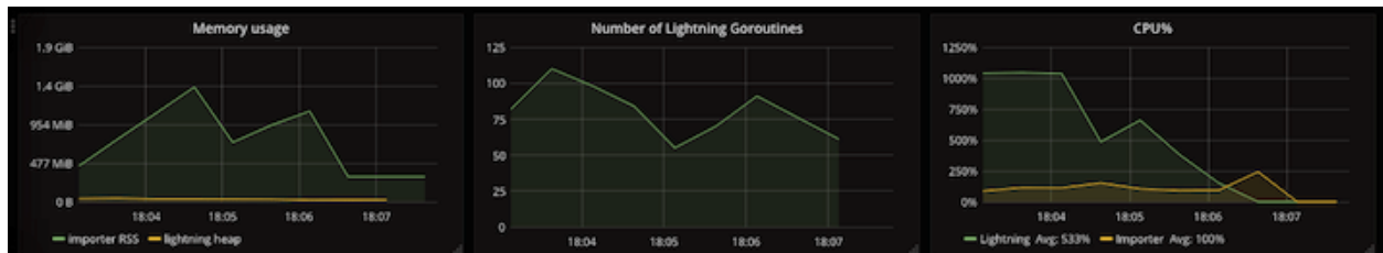
图 131: 第三行资源使用面板
