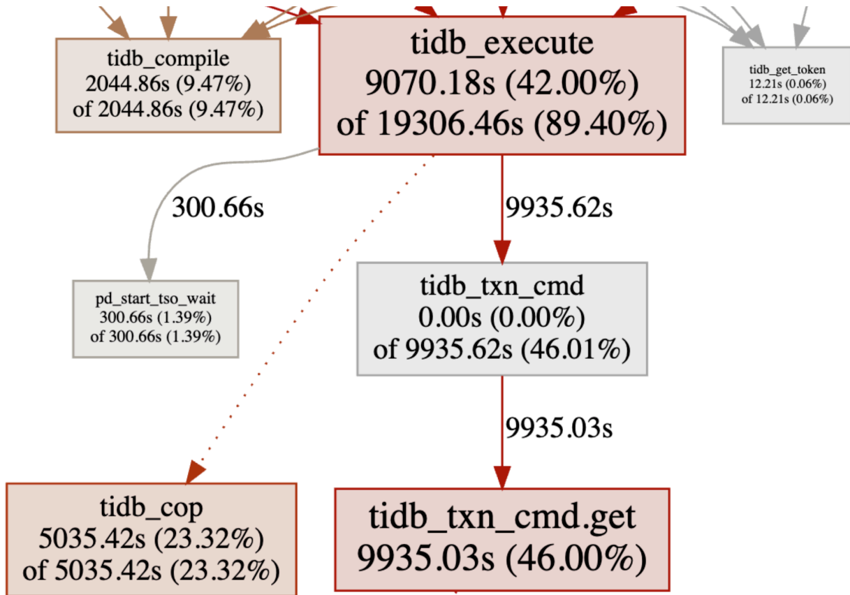
图 385: 监控关系图 tidb_execute 节点注释
