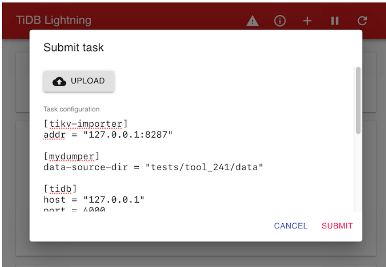
图 125: 提交任务对话框
