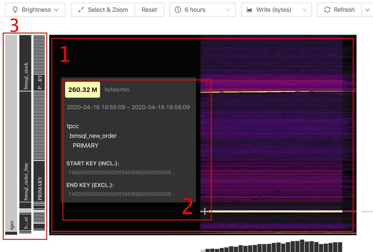
图 366: Key Visualizer 示例图
