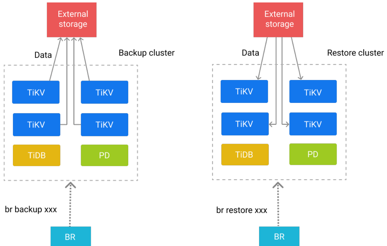
图 137: br-arch
