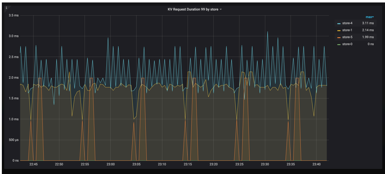
图 40: TiKV 相应时间
