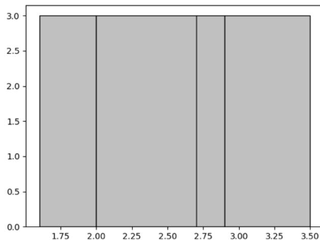
图 70: 等深直方图示例
