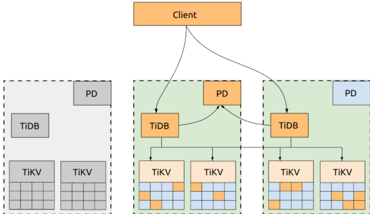
图 169: 三 AZ 部署容灾
