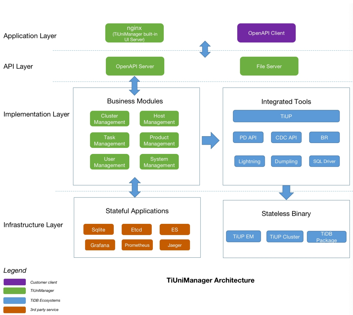
图 295: TiUniManager 架构图
