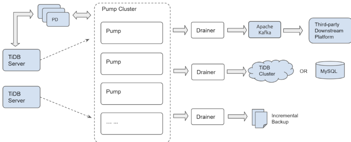
图 280: TiDB Binlog 架构
