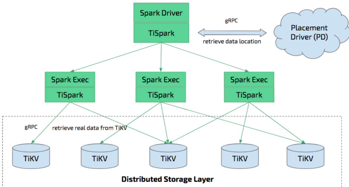
图 288: TiSpark 架构
