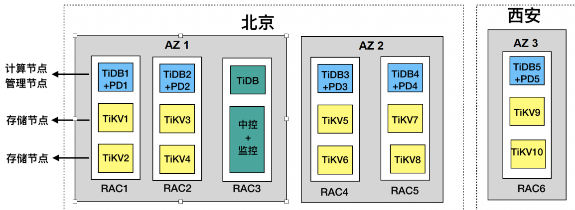
图 173: 双区域三 AZ 配置详图
