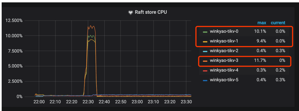
图 181: QPS3
