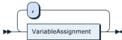
图 368: VariableAssignmentList
