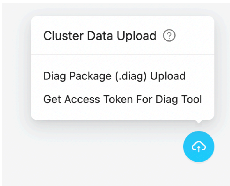
图 284: Token 示例
