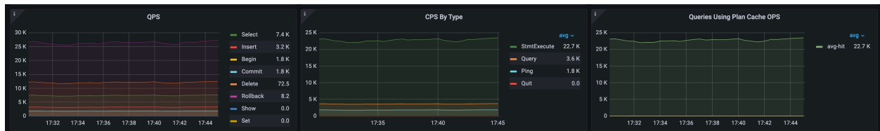
图 88: TPC-C
