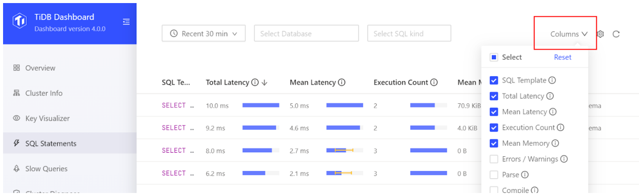
图 529: 选择列
