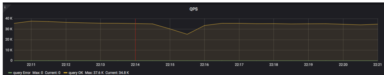
图 581: QPS 图
