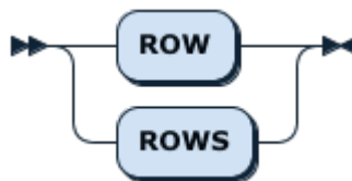
图 361: RowOrRows
