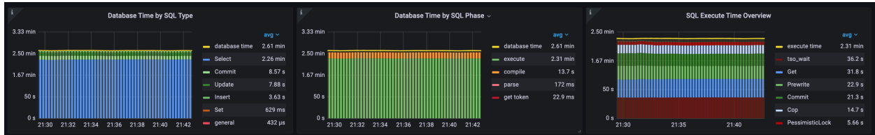
图 84: OLTP
