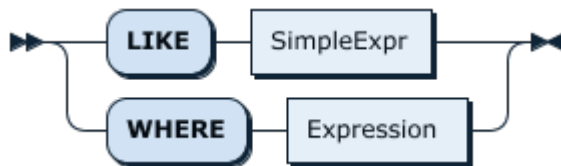
图 160: ShowLikeOrWhereOpt
