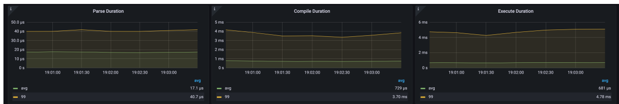
图 99: Compile
