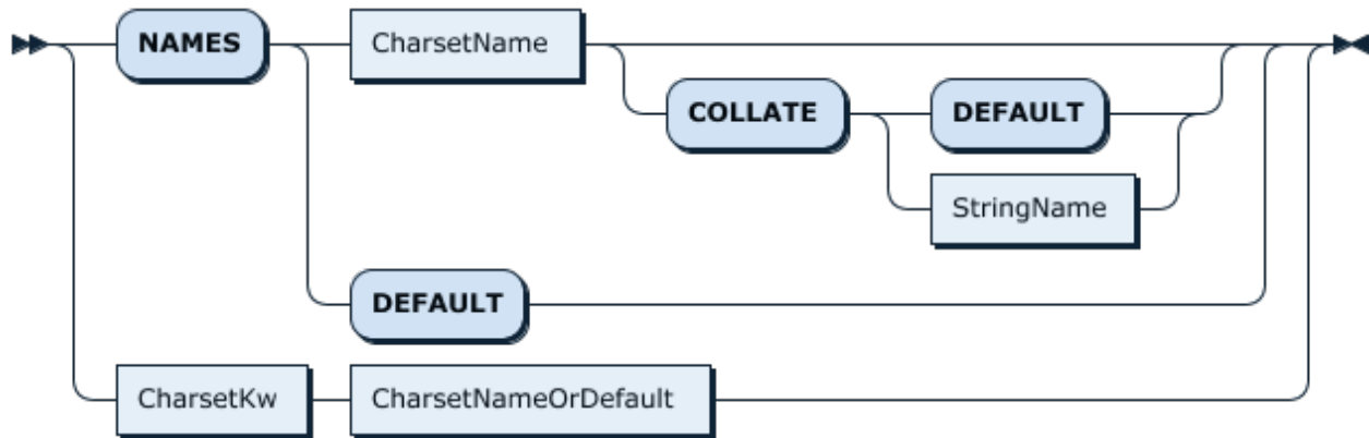
图 379: VariableAssignment
