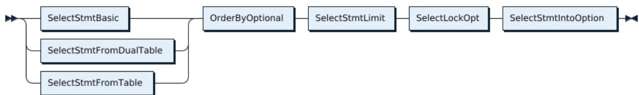
图 350: SelectStmt
