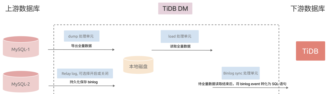
图 18: dm
