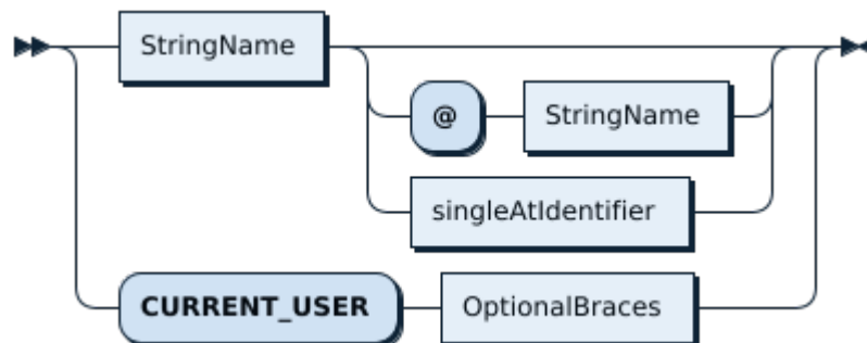
图 411: Username
