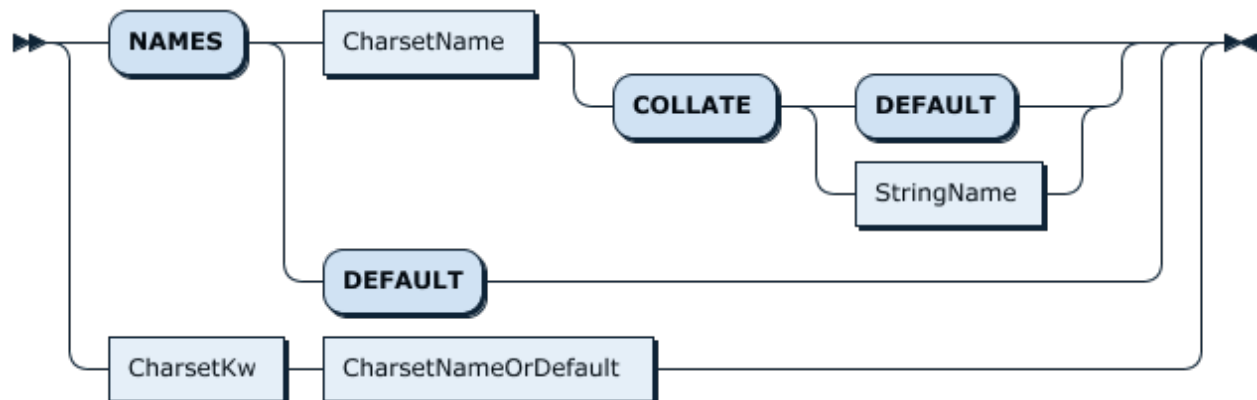
图 369: VariableAssignment
