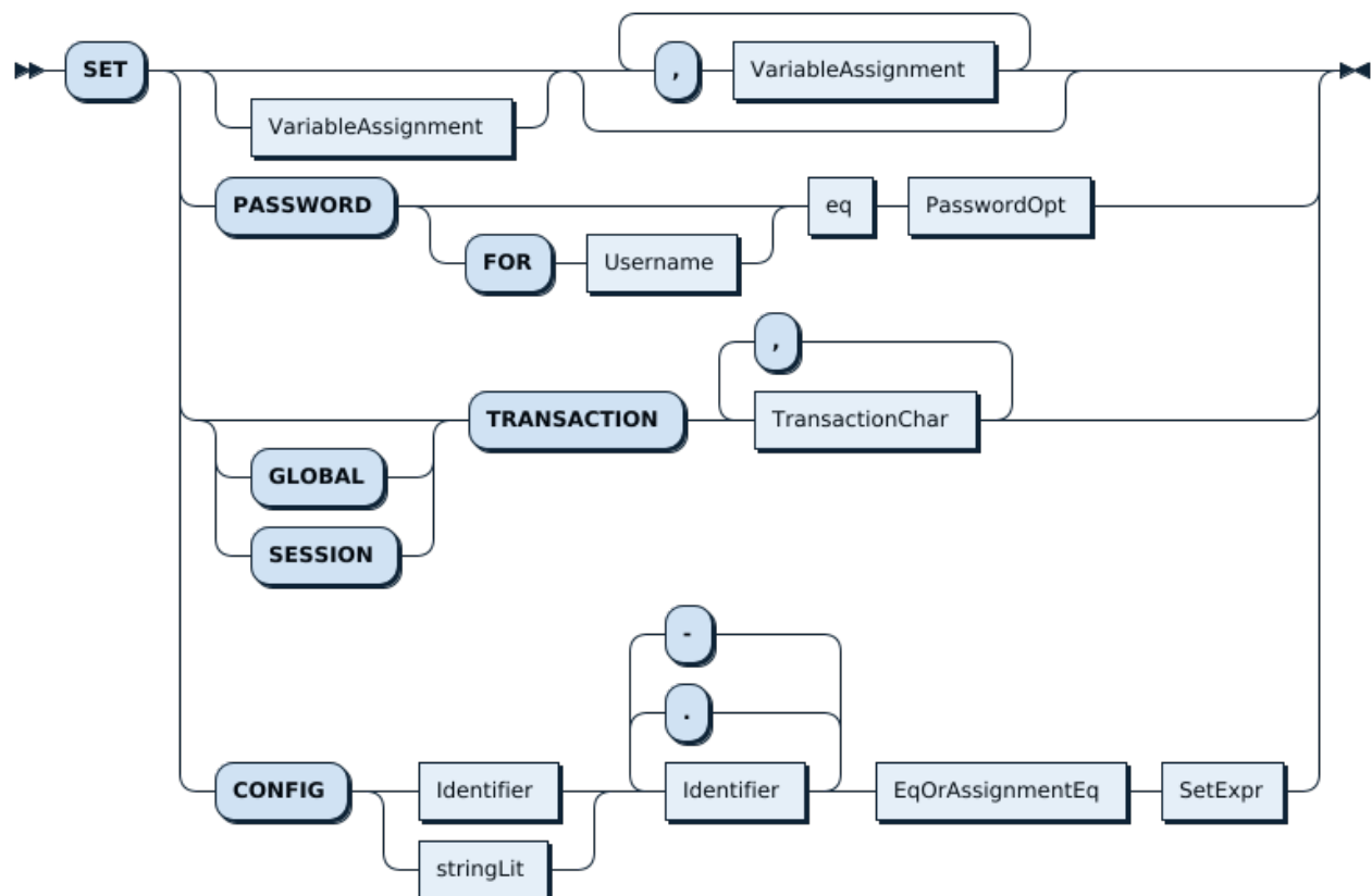
图 378: SetStmt
