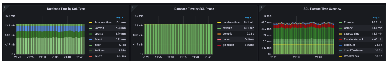
图 83: TPC-C
