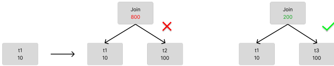
图 156: join-reorder-2
