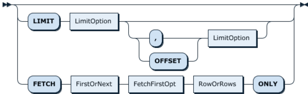
图 358: SelectStmtLimit
