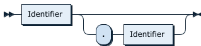
图 459: TableName
