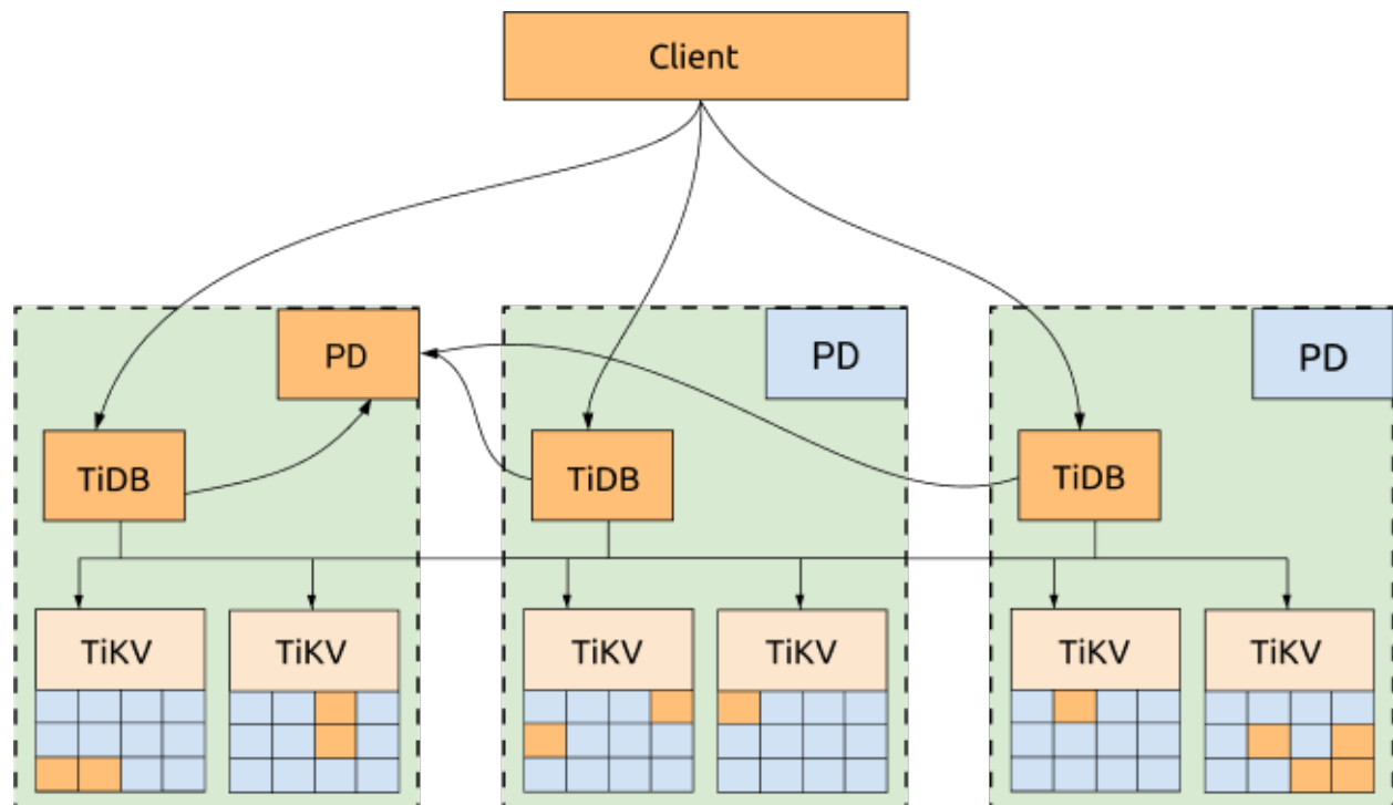
图 168: 三 AZ 部署
