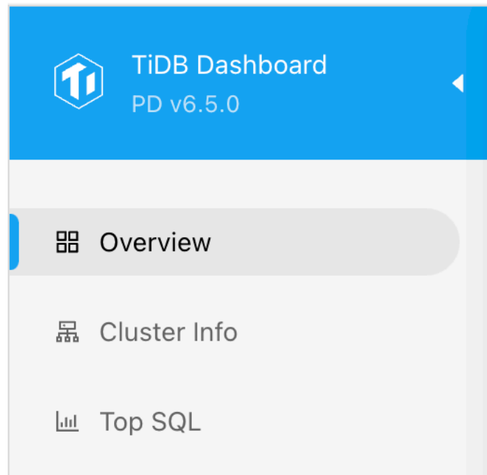
图 490: 访问
