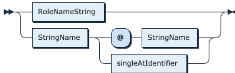
图 414: Rolename
