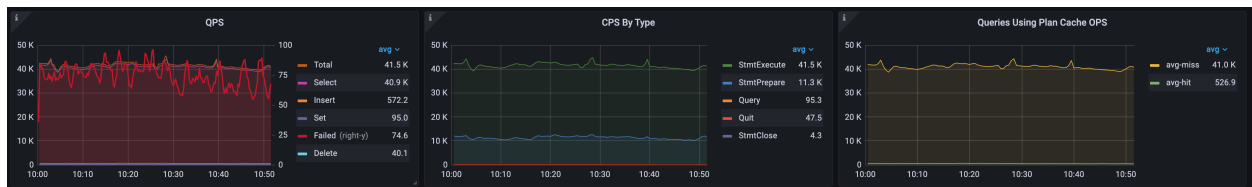
图 91: OLTP-Query
