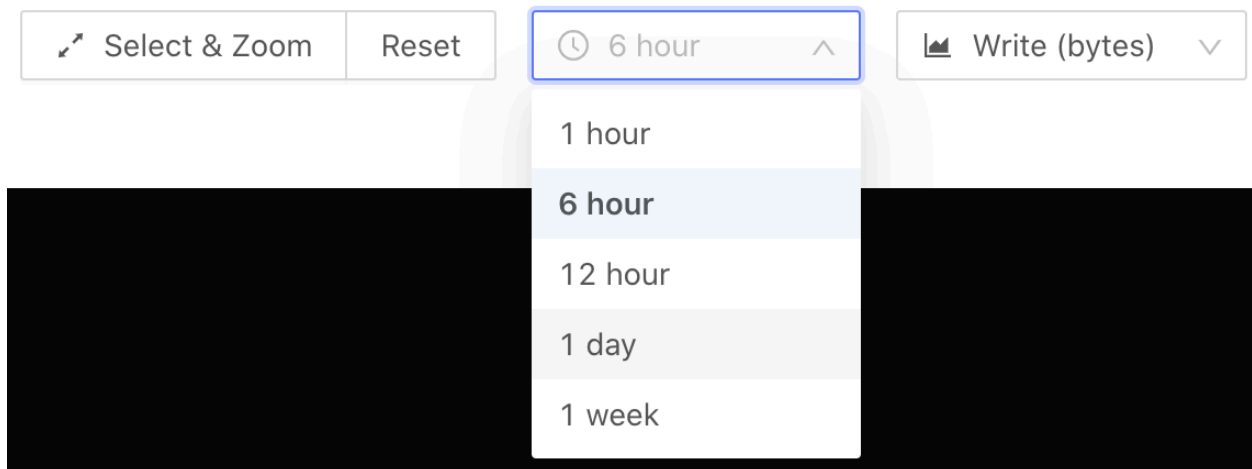
图 513: 时间选择
