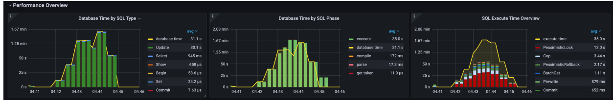
图 86: OLTP
