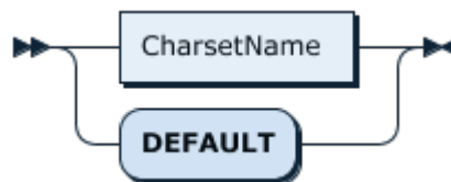
图 373: CharsetNameOrDefault
