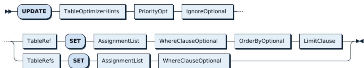
图 471: UpdateStmt
