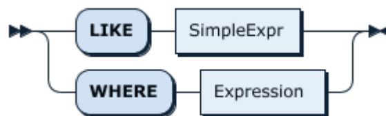
图 419: ShowLikeOrWhereOpt
