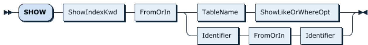
图 415: ShowIndexStmt
