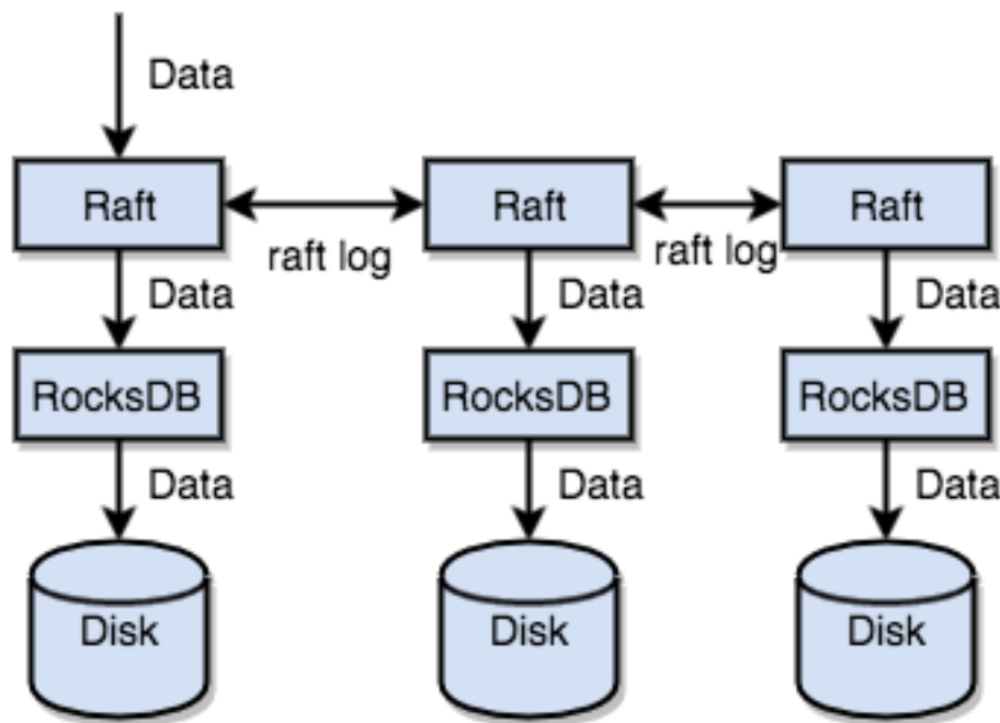
图 317: Raft in TiDB
