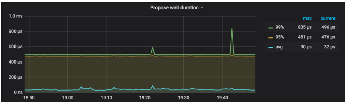
图 229: 图 3 查看 Propose wait duration
