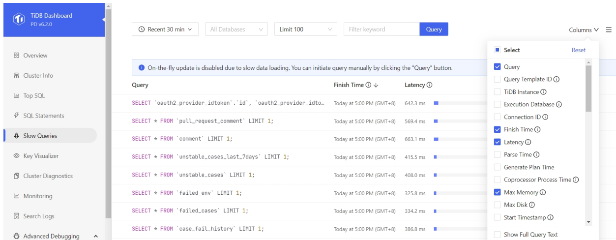
图 569: 显示更多列信息
