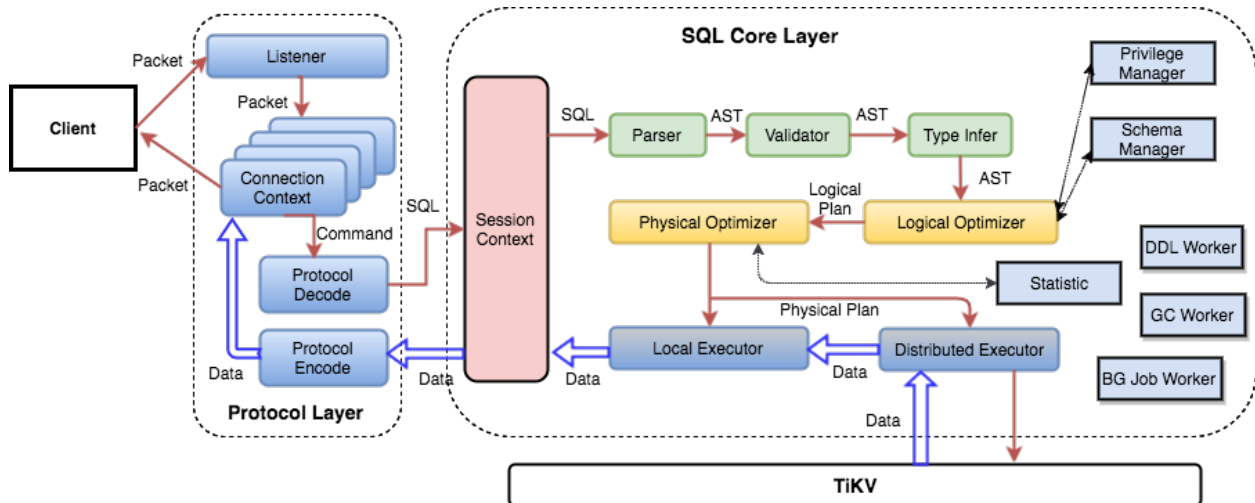
图 322: tidb sql layer
