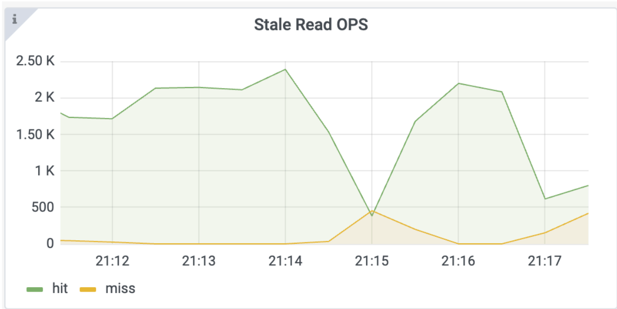
图 101: Example: Stale Read OPS
