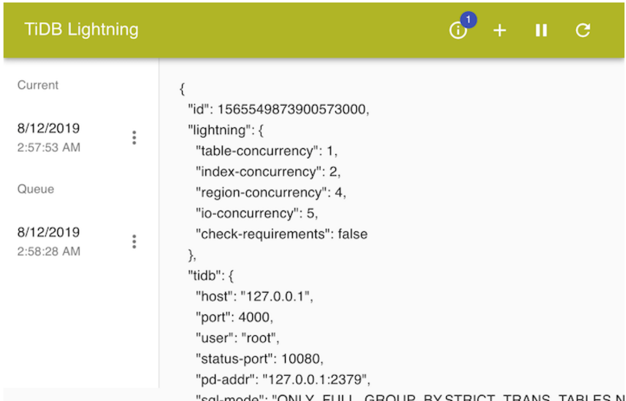
图 275: 任务管理页面
