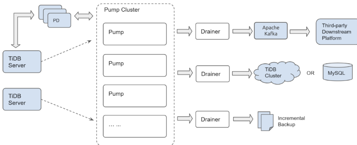
图 304: TiDB Binlog 架构
