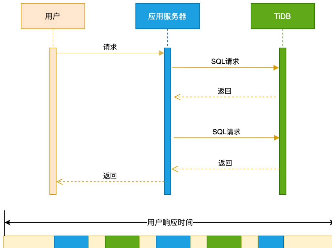
图 103: 用户响应时间
