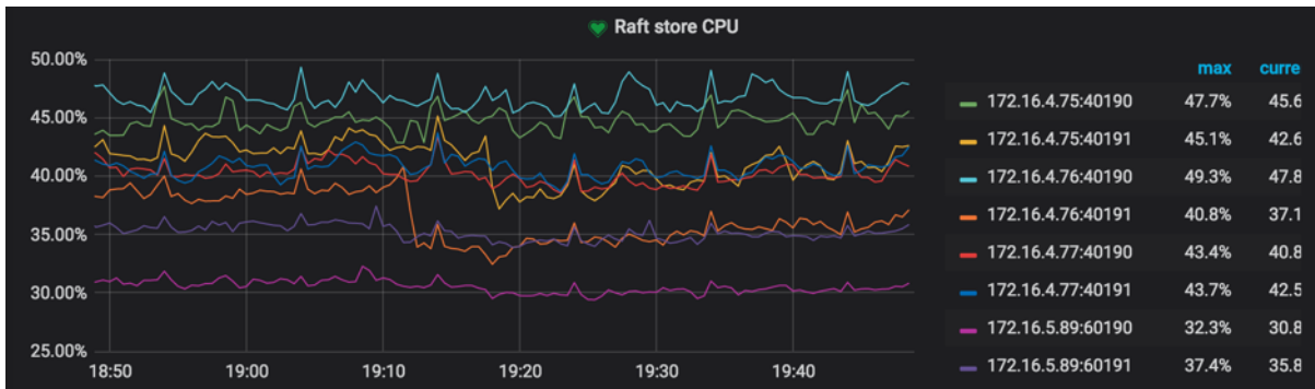
图 228: 图 2 查看 Raftstore CPU
