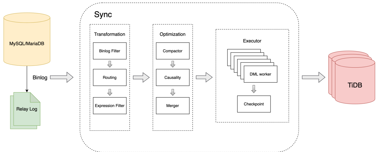
图 261: DML 处理逻辑
