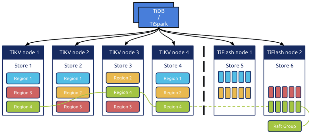
图 55: TiDB architecture
