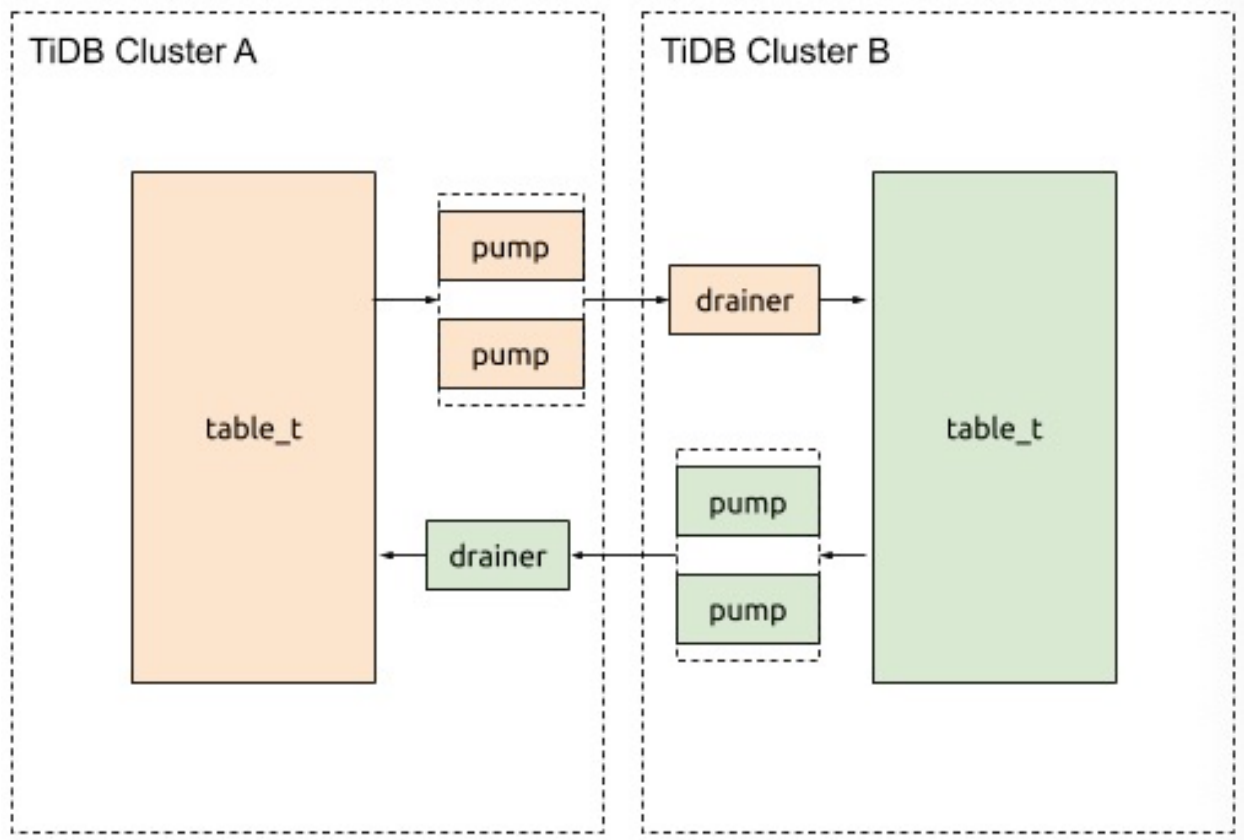
图 306: 使用场景示例图
