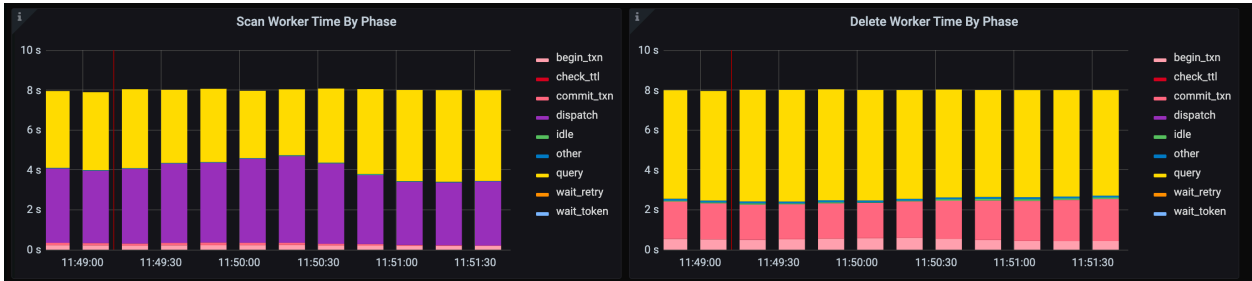
图 19: scan fast example
