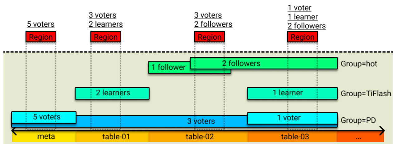
图 237: Placement rules overview
