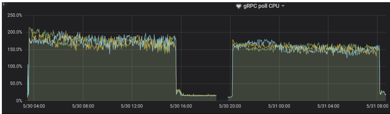
图 233: gRPC Pool CPU
