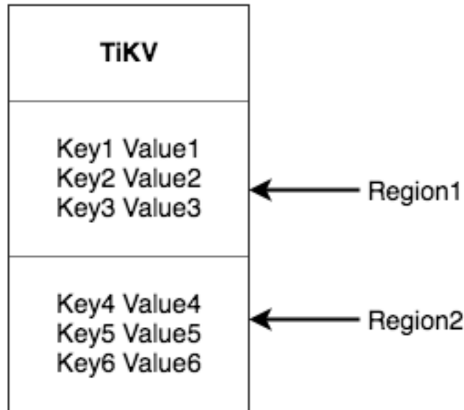
图 318: Region in TiDB
