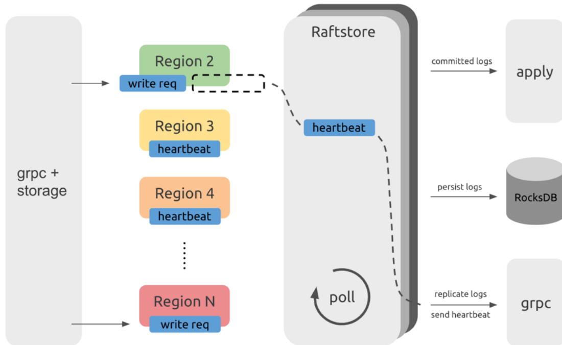
图 227: 图 1 Raftstore 处理流程示意图
