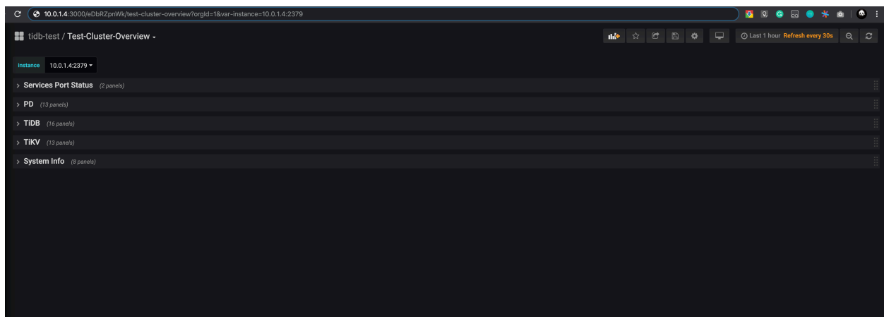
Figure 93: Grafana-overview
