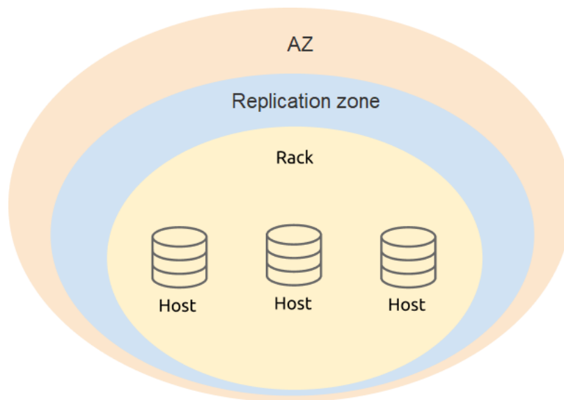
图 202: Label 逻辑定义图
