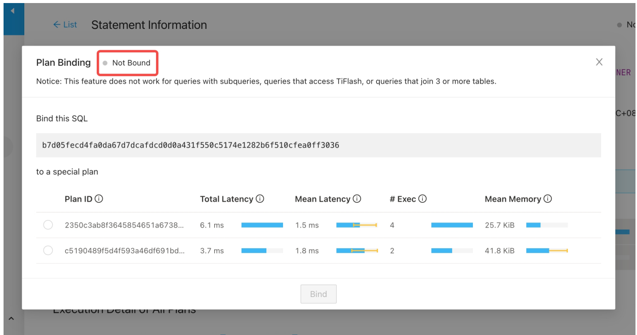
图 445: 快速绑定执行计划 -弹窗
