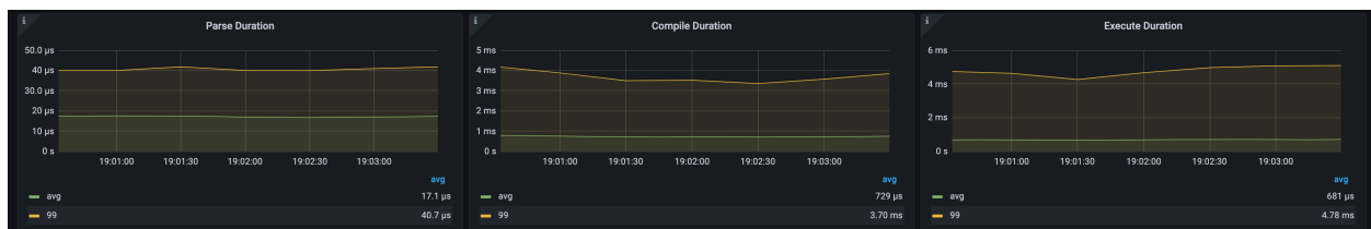
图 129: Compile
