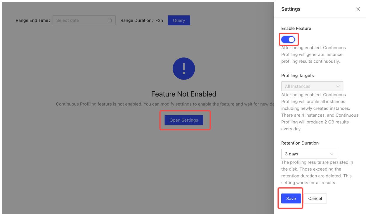
图 516: 启用功能
