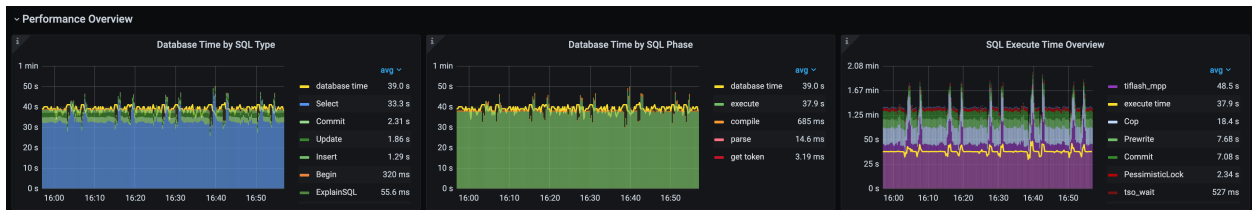
图 114: HTAP
