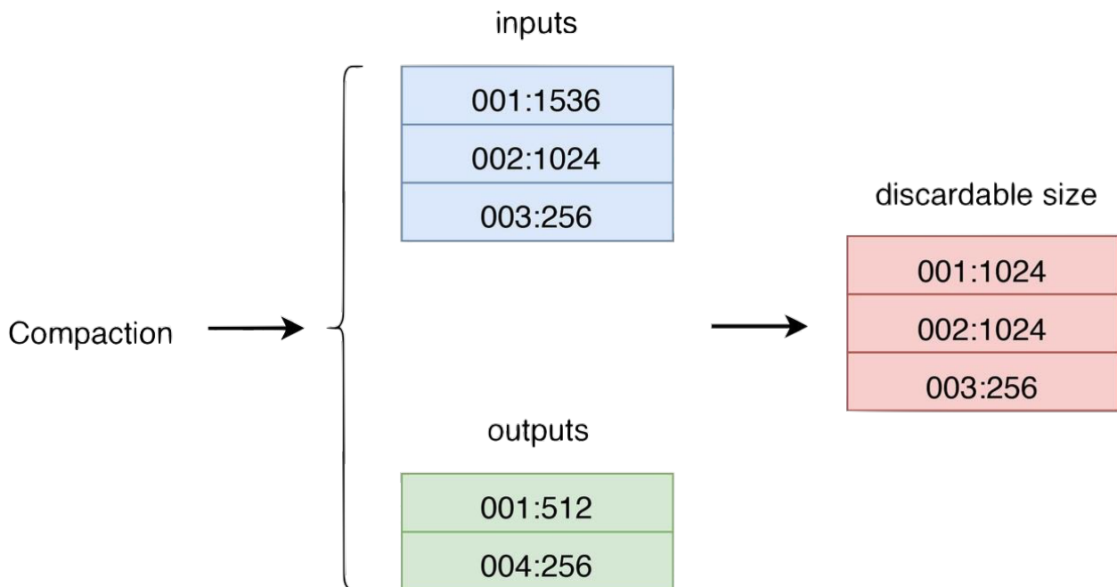
图 338: EventListener
