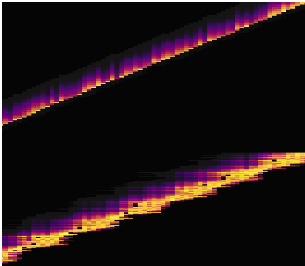
图 425: 明亮斜线
