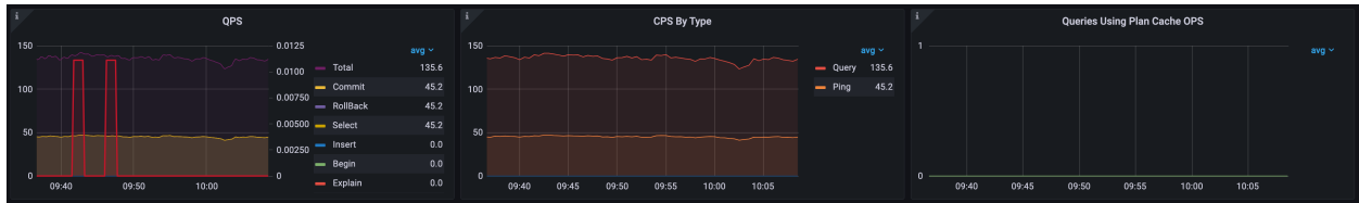
图 116: OLTP-Query
