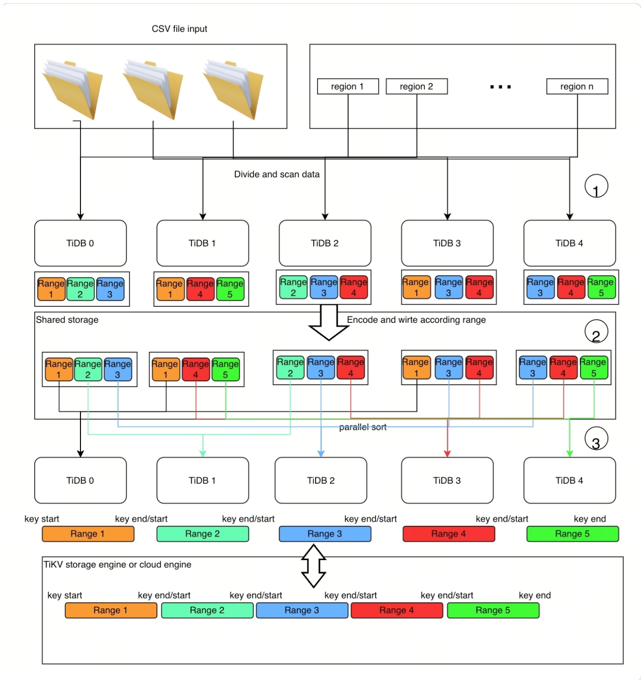
图 348: 全局排序功能算法
