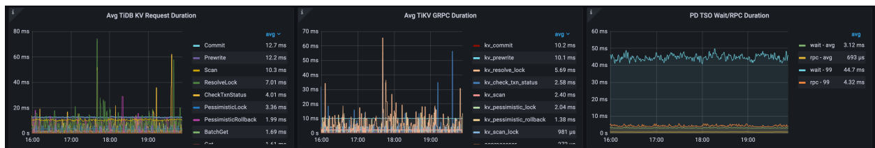
图 133: Cloud Env
