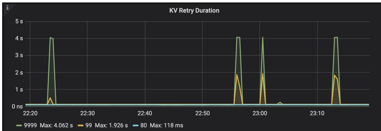
图 95: kv-retry-duration
