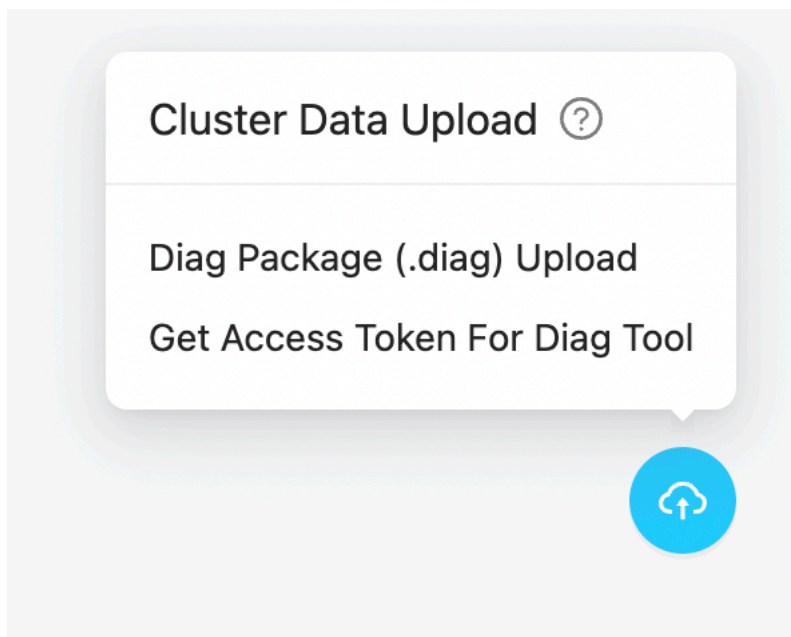
图 317: Token 示例
