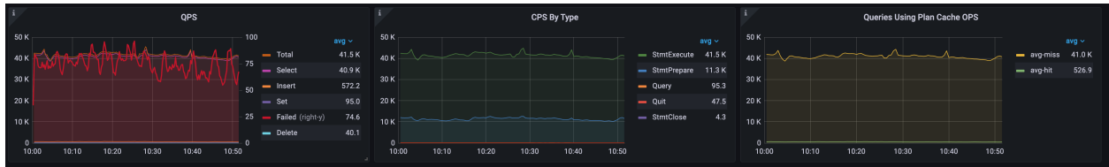
图 118: OLTP-Query
