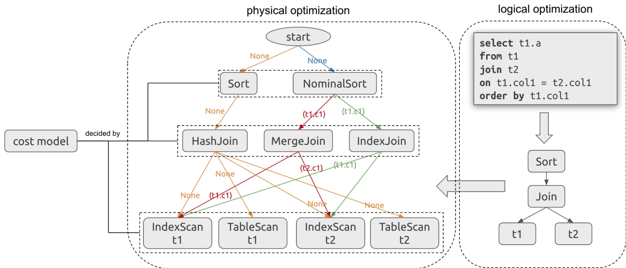
图 191: CostModel
