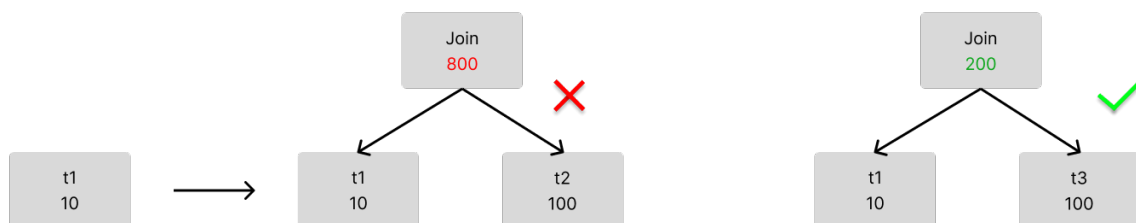
图 186: join-reorder-2
