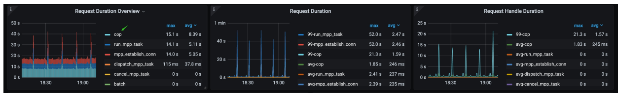
图 175: Cop
