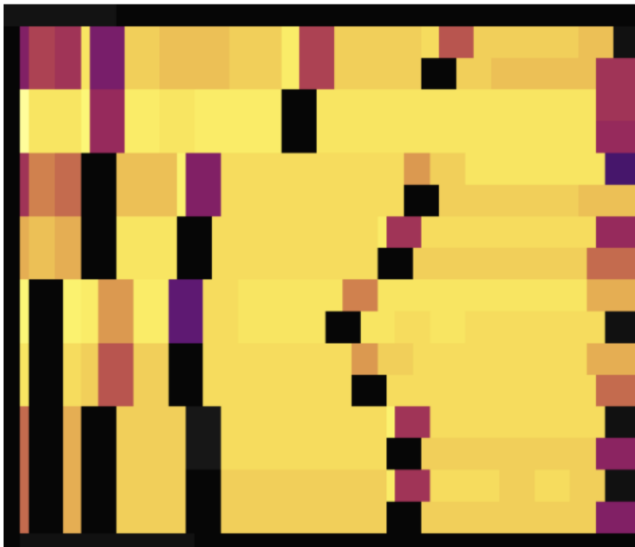
图 90: Dashboard 示例 6
