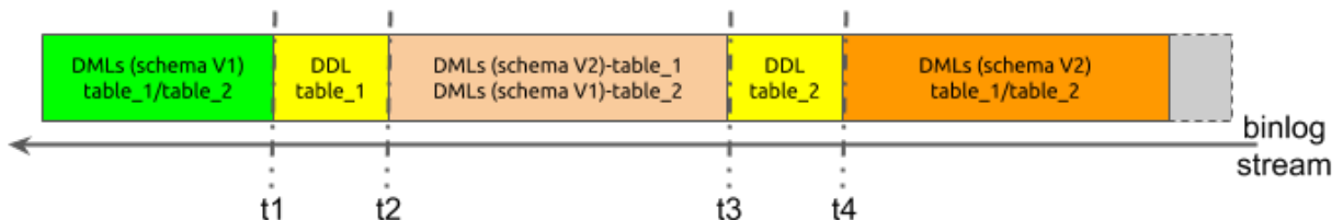
图 248: shard-ddl-example-2
