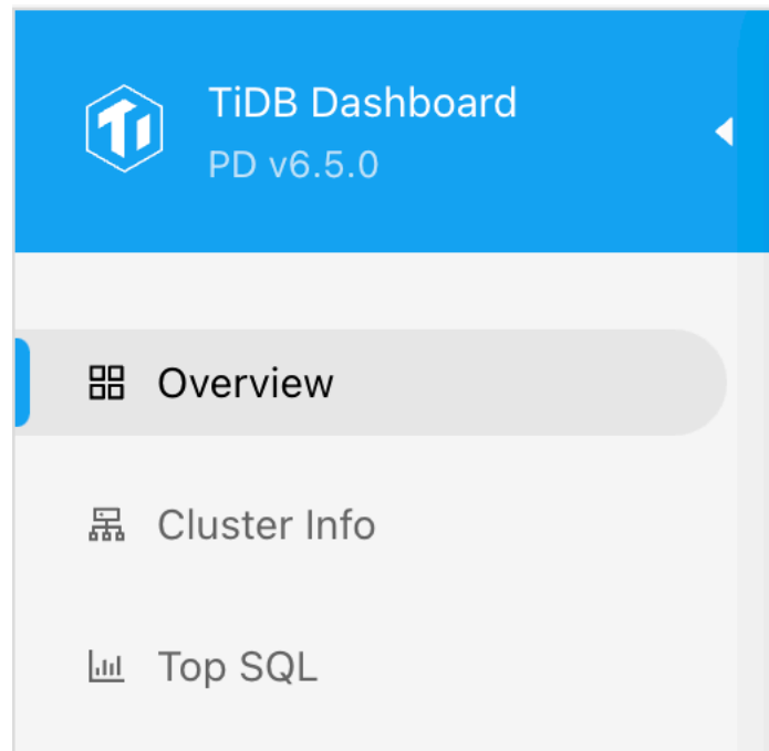
图 395: 访问
