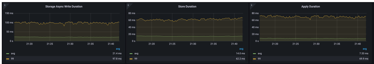
图 137: v5.4.0
