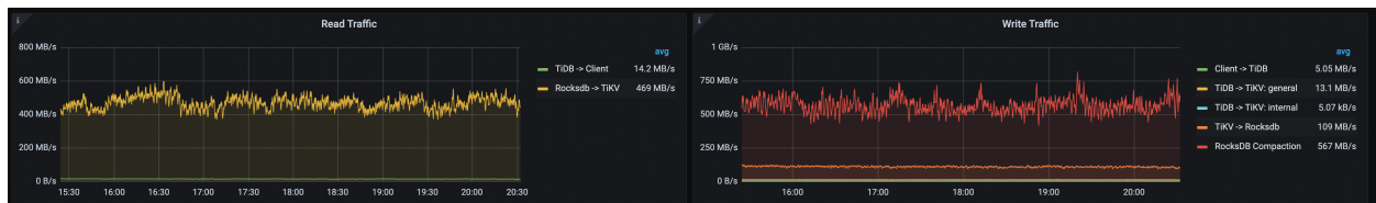
图 122: TPC-C
