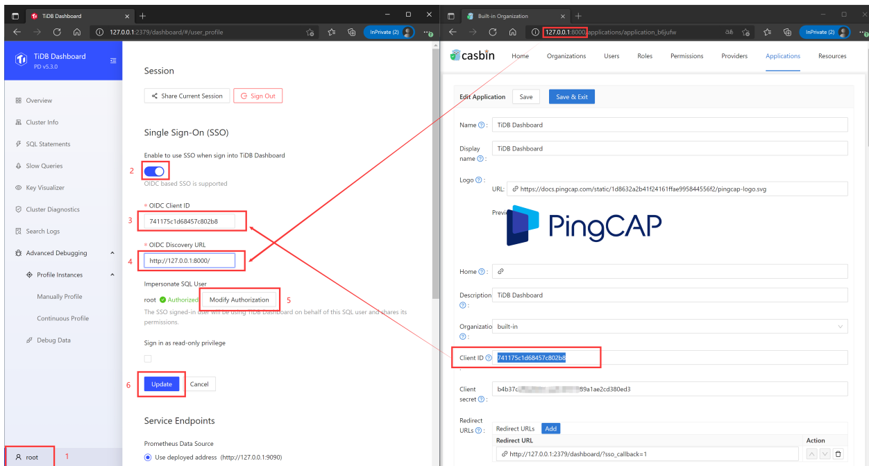
图 546: Settings
