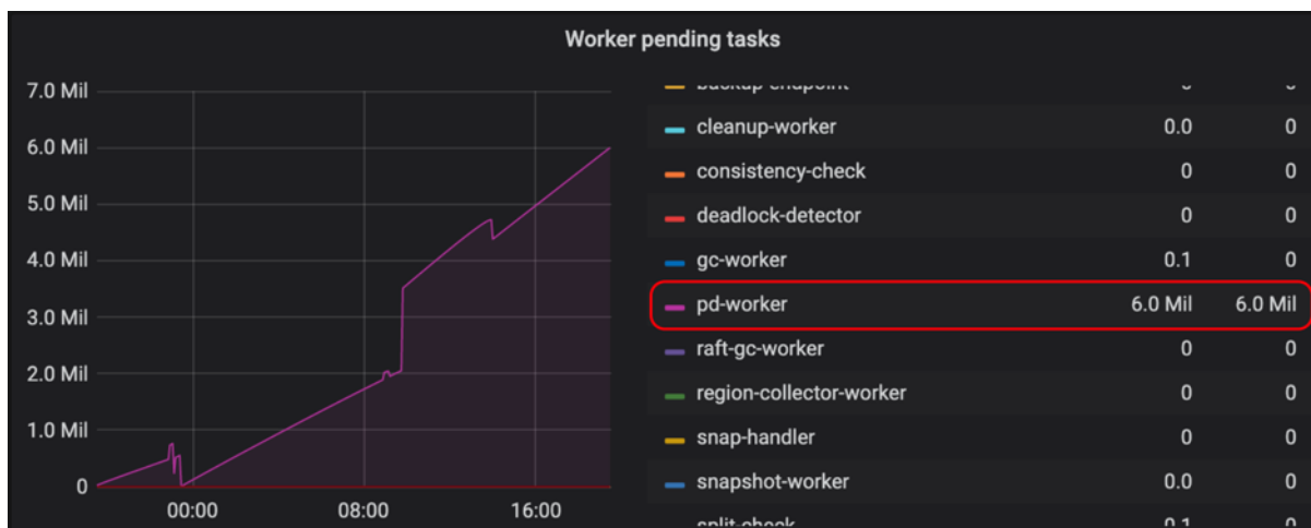
图 236: 图 4 查看 pd-worker
